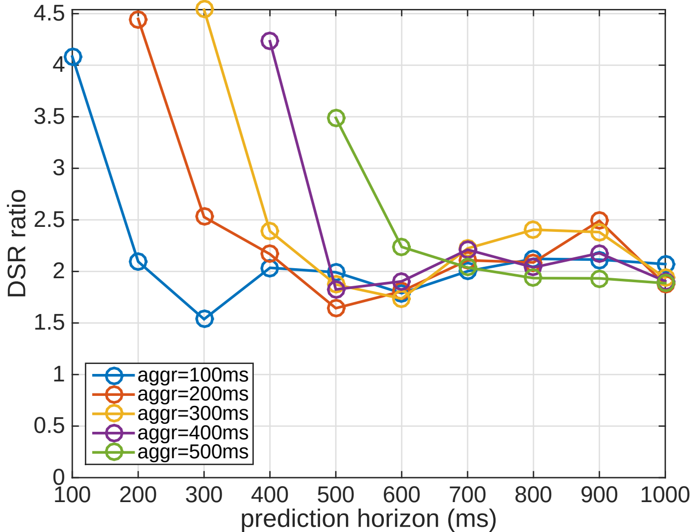
error Baseline / error NN
