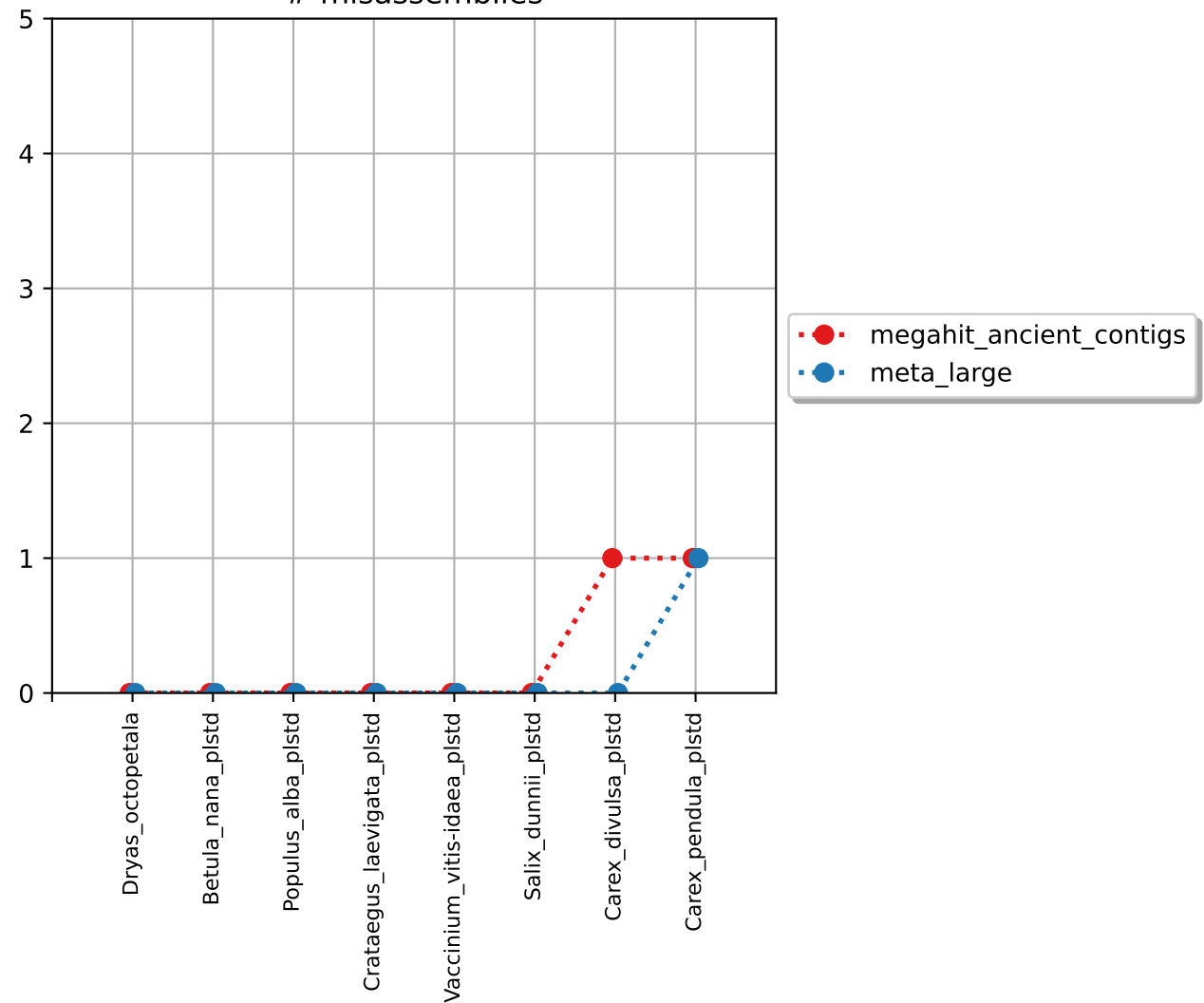
# misassemblies
