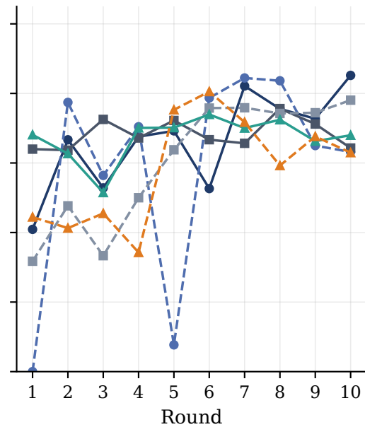
F1
