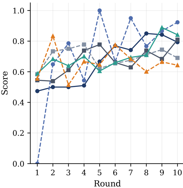
Precision
