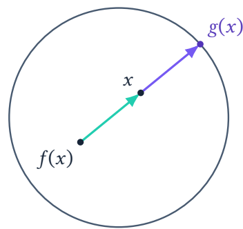
B^2 : круг вместе с границей
