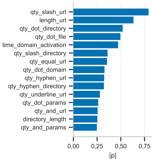
|Spearman| con la clase
