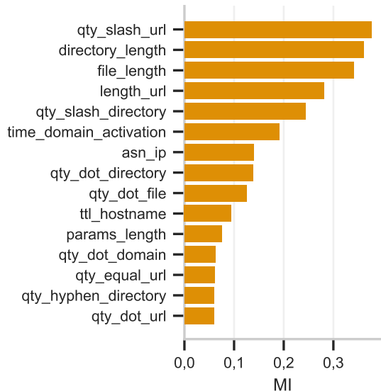
Información mutua con la clase
