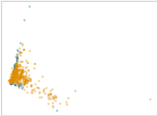
PCA (2 componentes)
