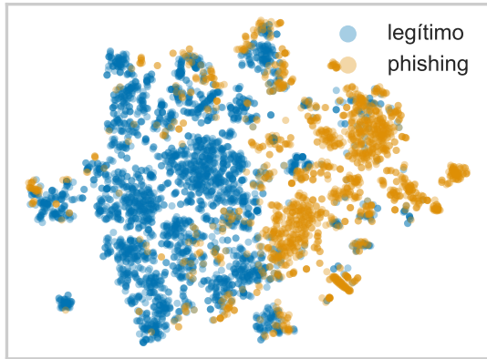
t-SNE (2 componentes)
