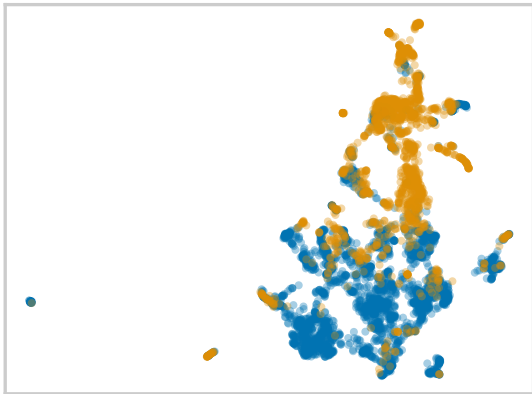
UMAP
