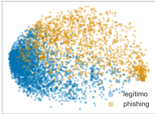
Kernel PCA (RBF)
