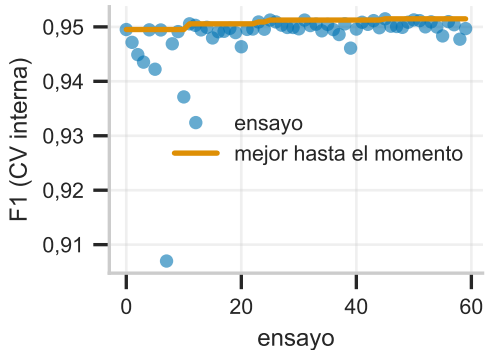
Convergencia de la búsqueda
