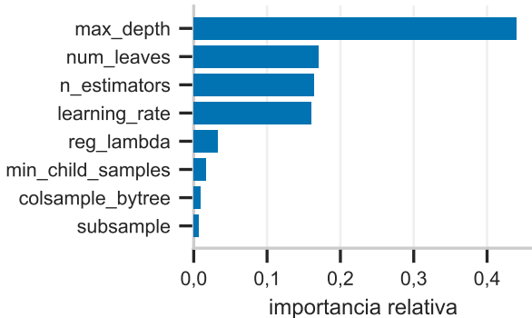
Qué hiperparámetros importan
