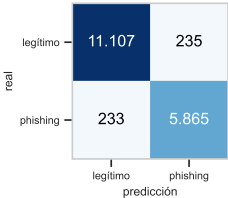
Matriz de confusión (recuentos)
