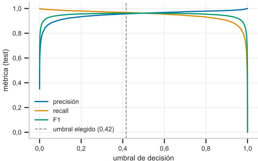
Precisión, recall y F1 según el umbral (test)
