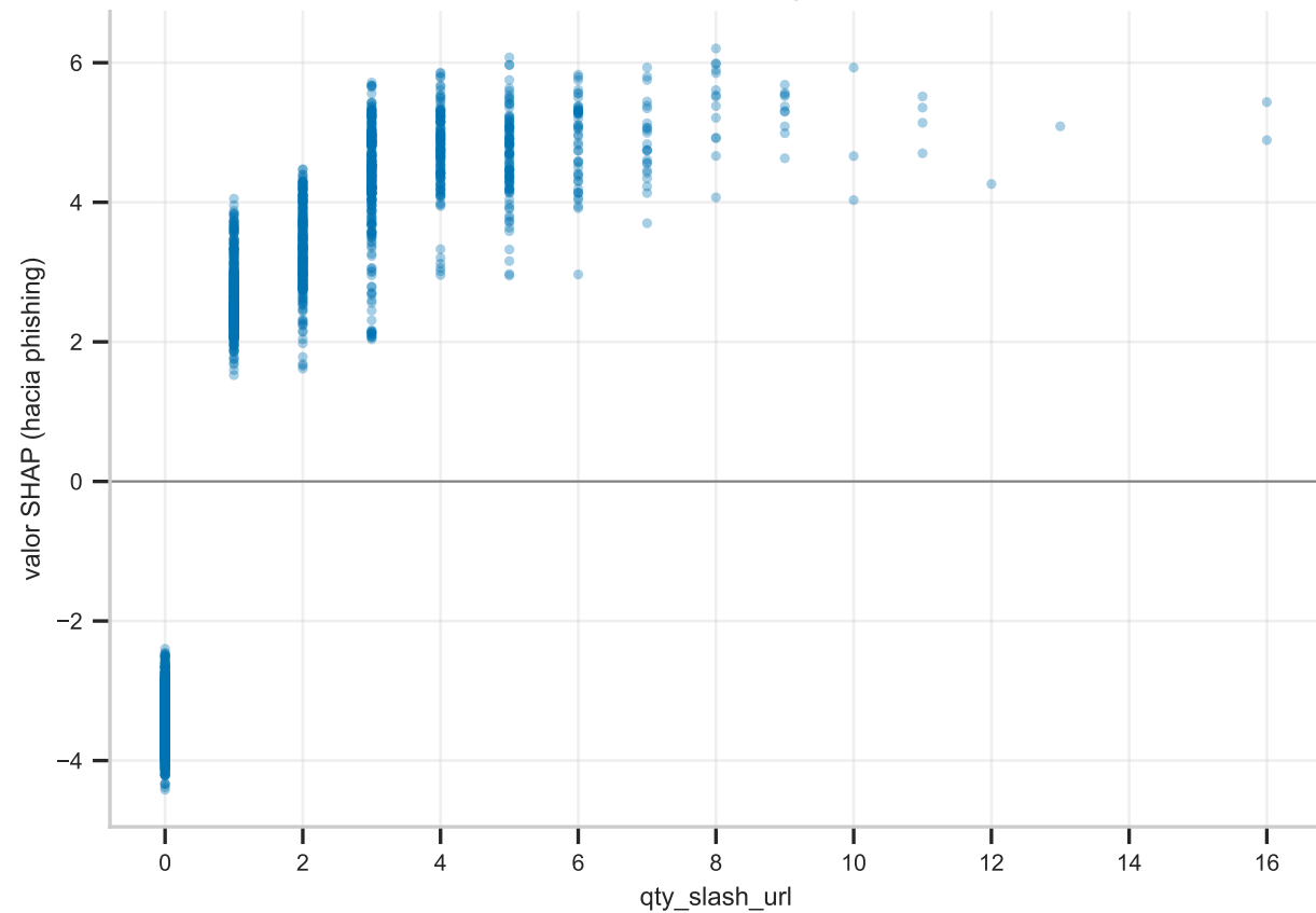
Dependencia SHAP: qty_slash_url
