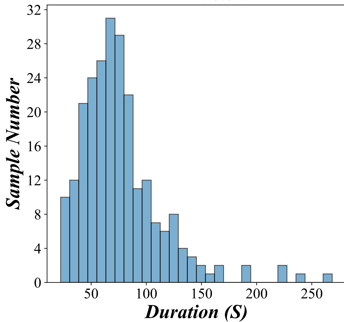
ADReSSo
