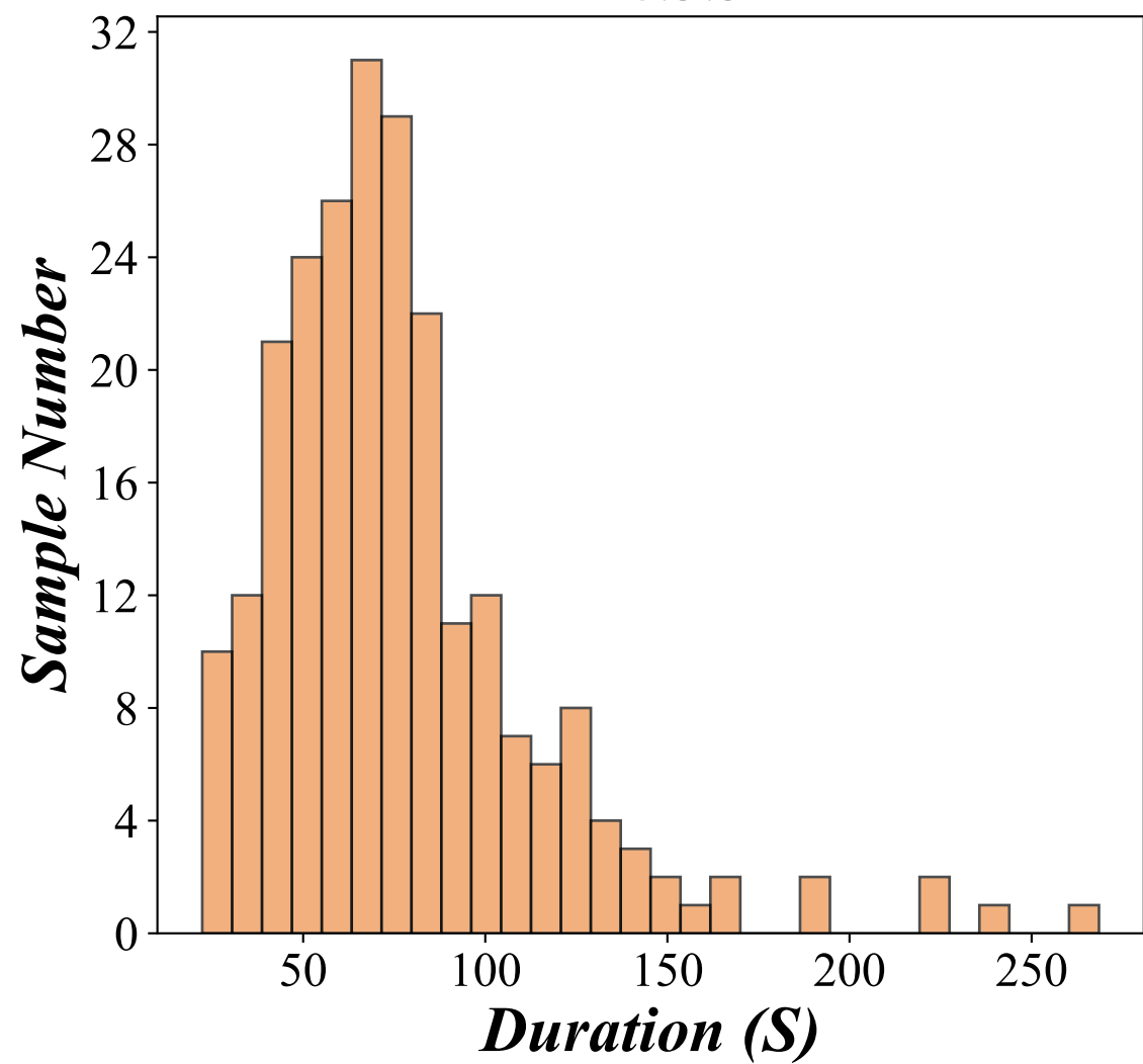
ADReSS-M
