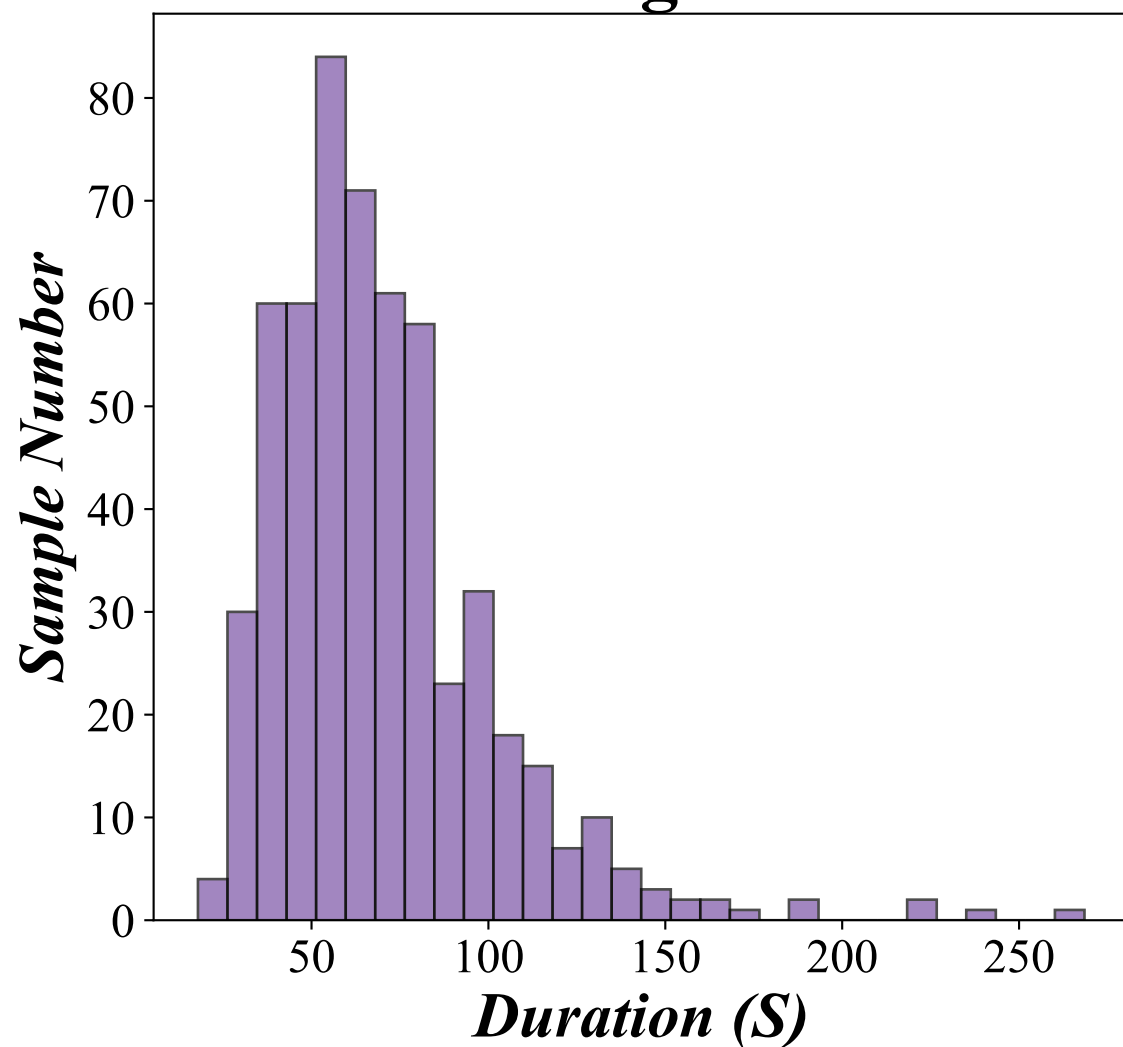
ADReSSo
