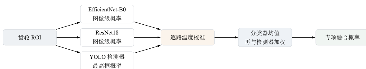
图2 单个专项模型包的融合方式
