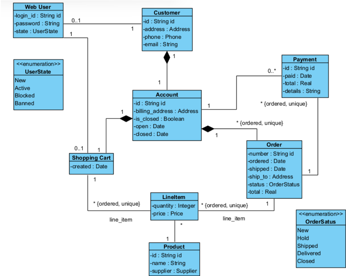
Диаграмма классов (Class Diagram)
