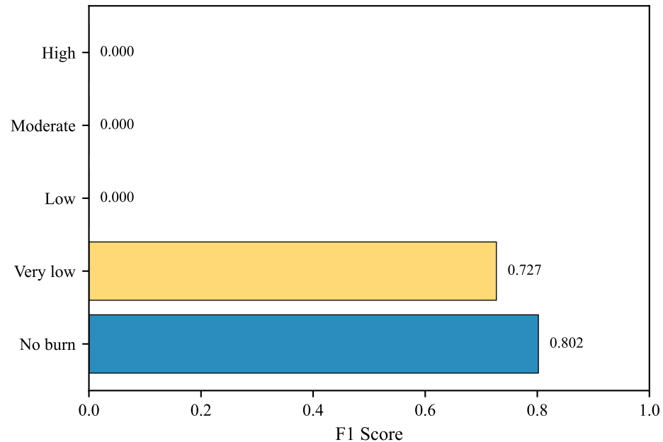
(b) Per-Class F1 Score
