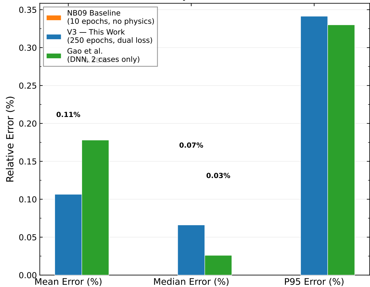
(d) Method Comparison — Error Metrics
