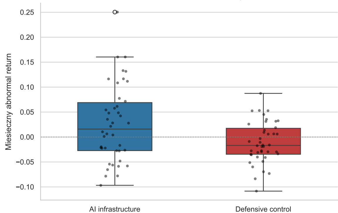
Zad 1 - boxplot porównawczy
