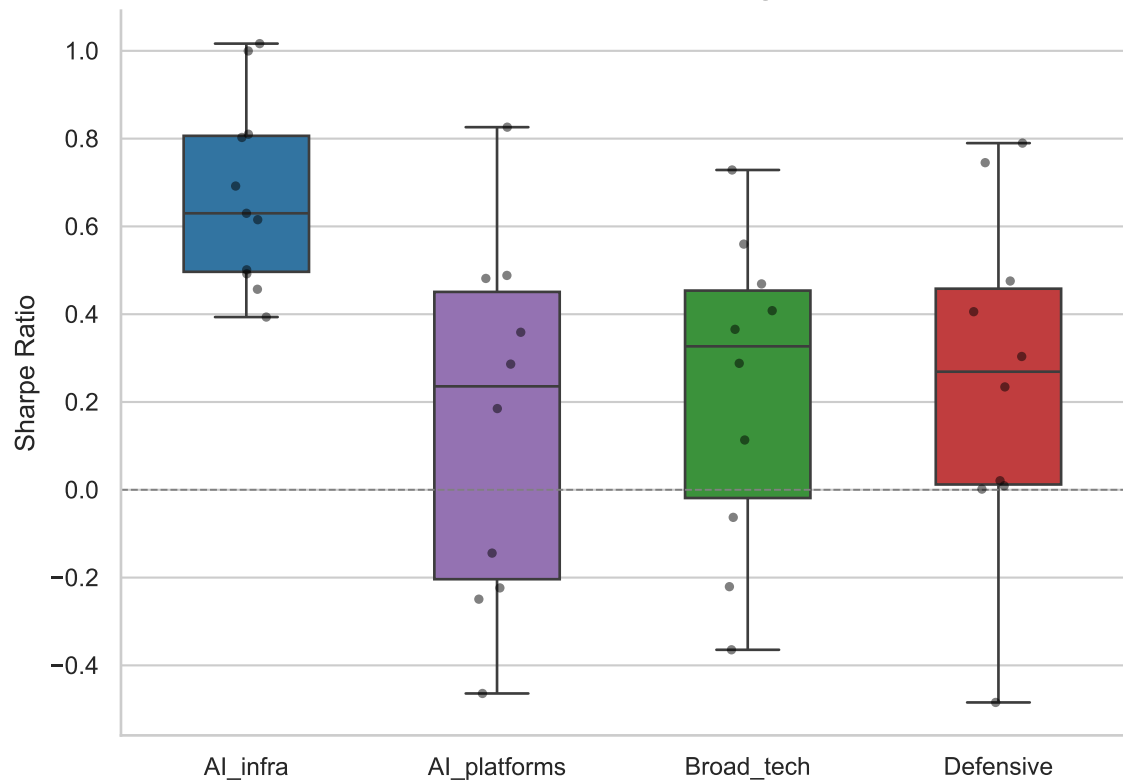
Boxplot - Sharpe Ratio per grupa
