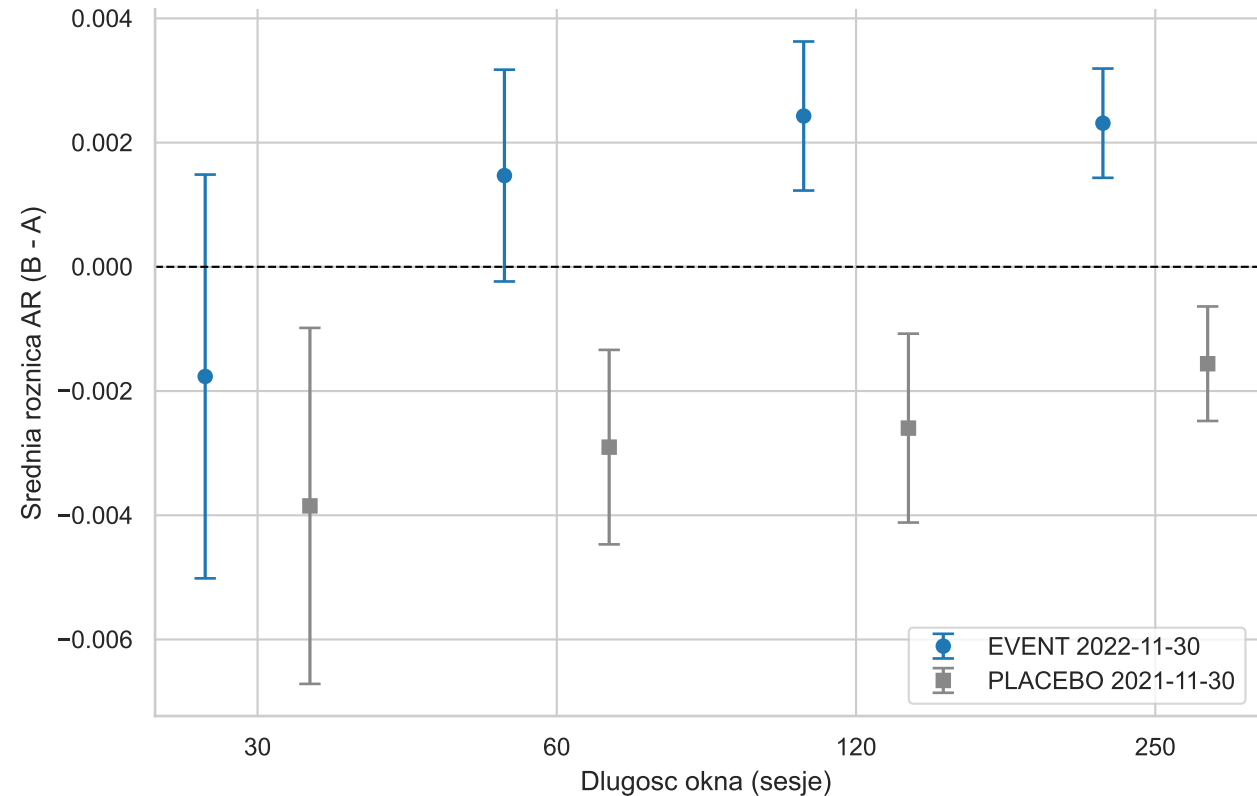
Analiza wzrazliwosci + placebo
