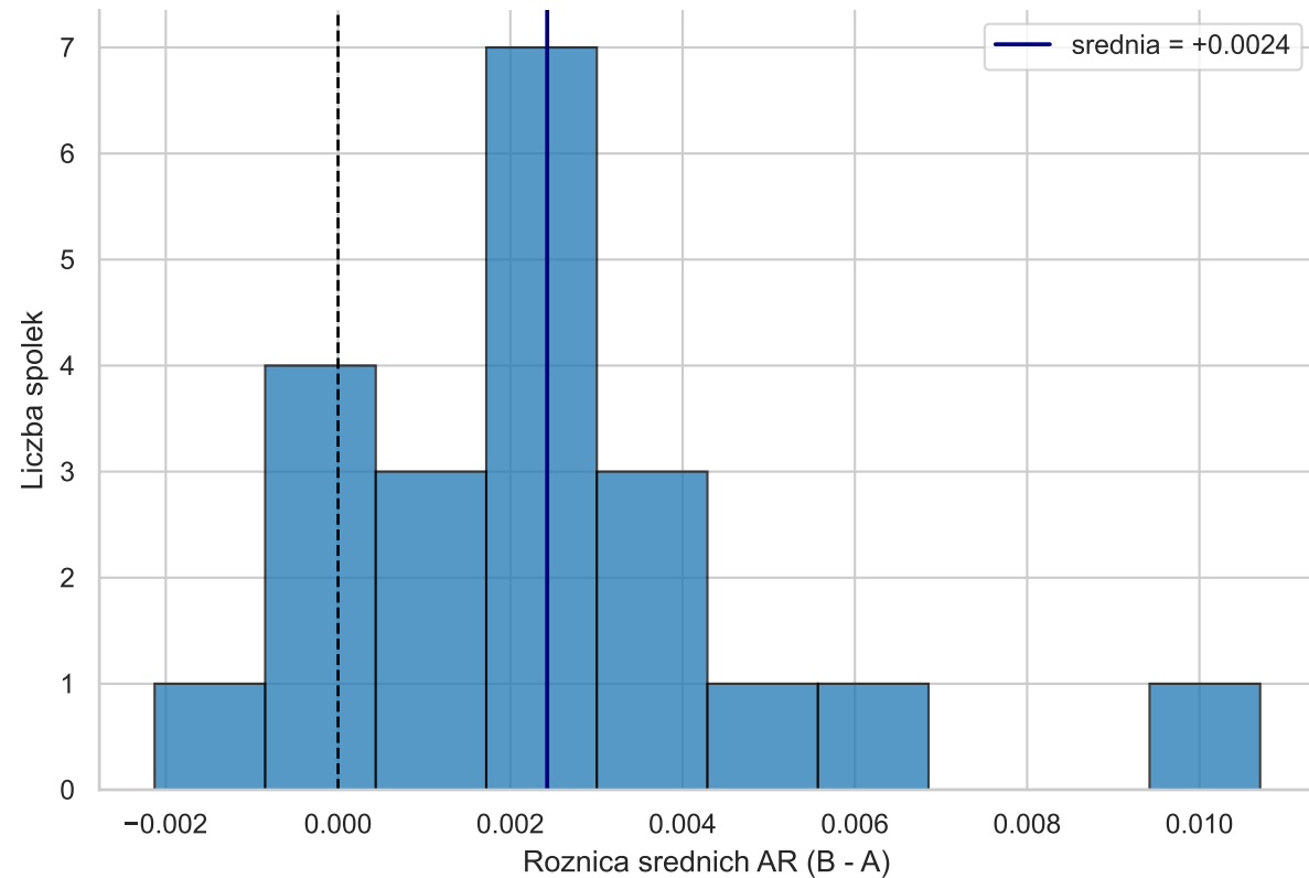
Histogram roznic - okno 120 sesji
