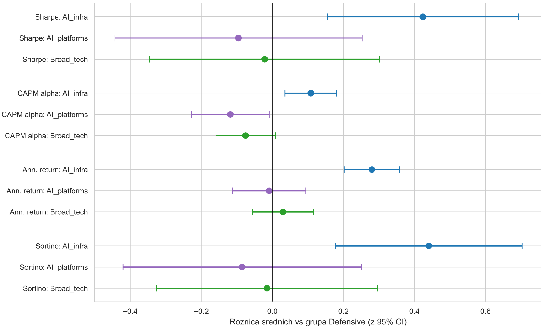
Forest plot - roznice metryk wzgledem grupy Defensive (baseline)
