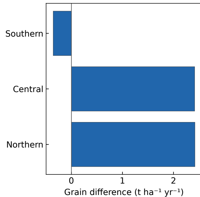
(f) Area-weighted latitude bands
