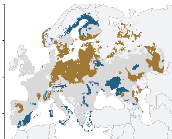
b SSP2-4.5 · 2031-2060
