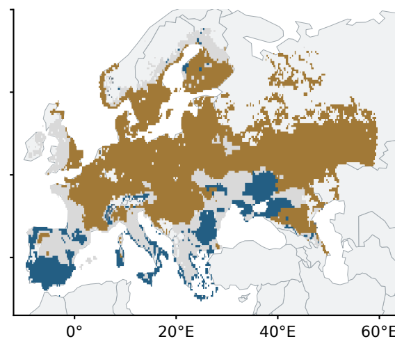
f SSP5-8.5 · 2071-2100
