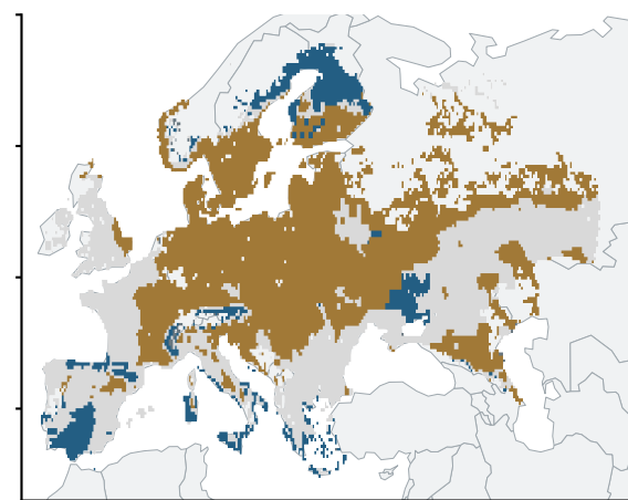
c SSP5-8.5 · 2031-2060
