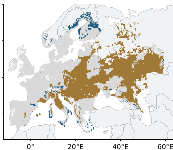
d SSP1-2.6 · 2071-2100
