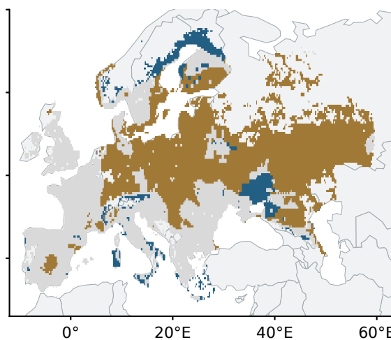
e SSP2-4.5 · 2071-2100
