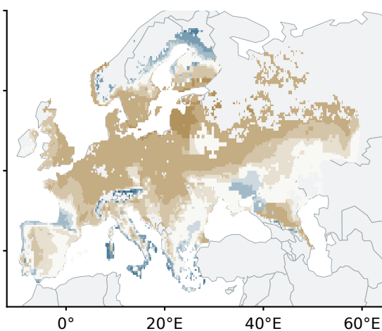
e SSP2-4.5 · 2071-2100
