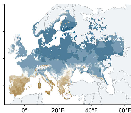
f SSP5-8.5 · 2071-2100
