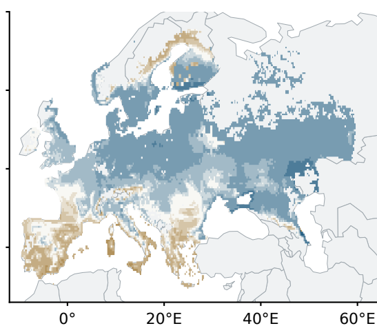
e SSP2-4.5 · 2071-2100
