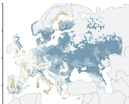
a SSP1-2.6 · 2031-2060
