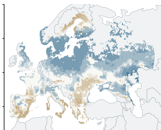
b SSP2-4.5 · 2031-2060
