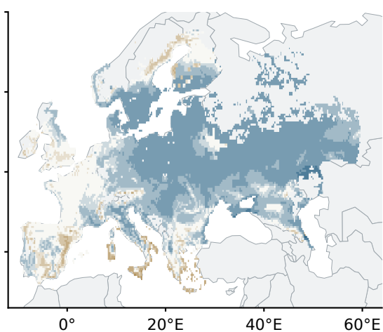
d SSP1-2.6 · 2071-2100
