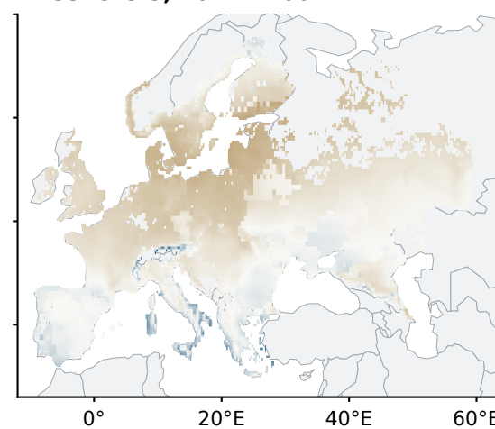
f SSP5-8.5; 2071-2100
