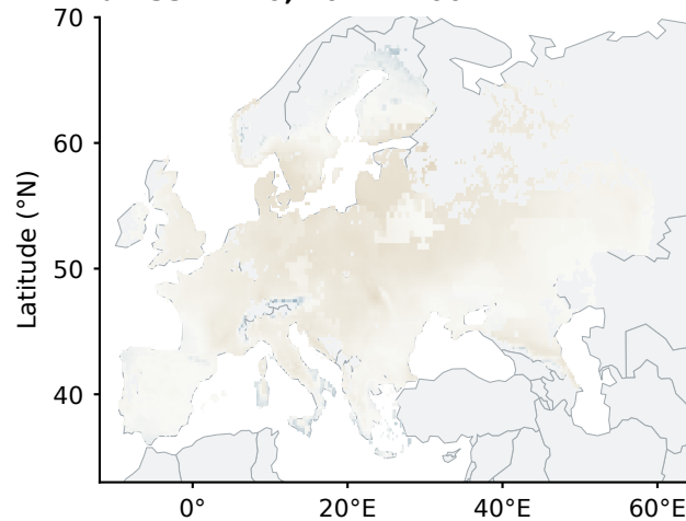
d SSP1-2.6; 2071-2100
