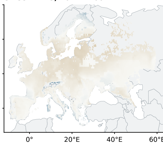
e SSP2-4.5; 2071-2100
