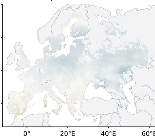
e SSP2-4.5; 2071-2100
