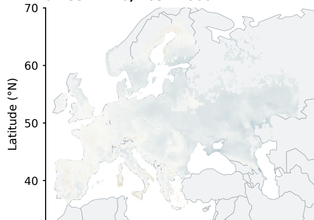
a SSP1-2.6; 2031-2060
