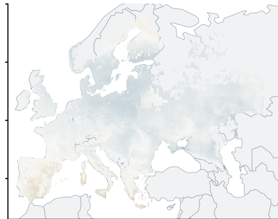
c SSP5-8.5; 2031-2060
