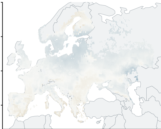
b SSP2-4.5; 2031-2060
