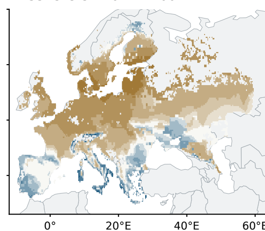
f SSP5-8.5 · 2071-2100
