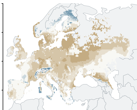
a SSP1-2.6 · 2031-2060
