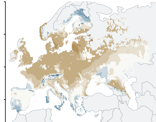
c SSP5-8.5 · 2031-2060
