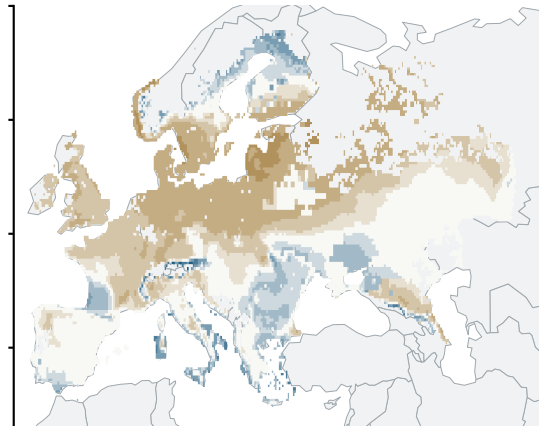
b SSP2-4.5 · 2031-2060
