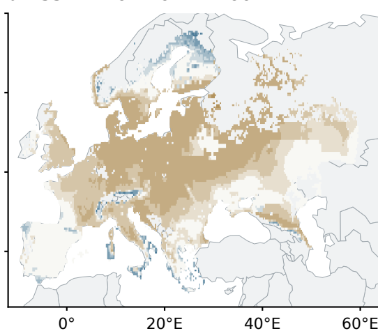
d SSP1-2.6 · 2071-2100
