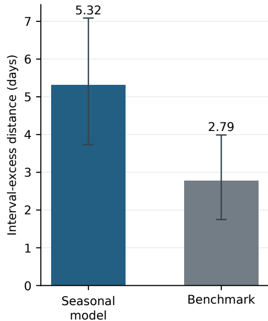
a Symptom-onset error
