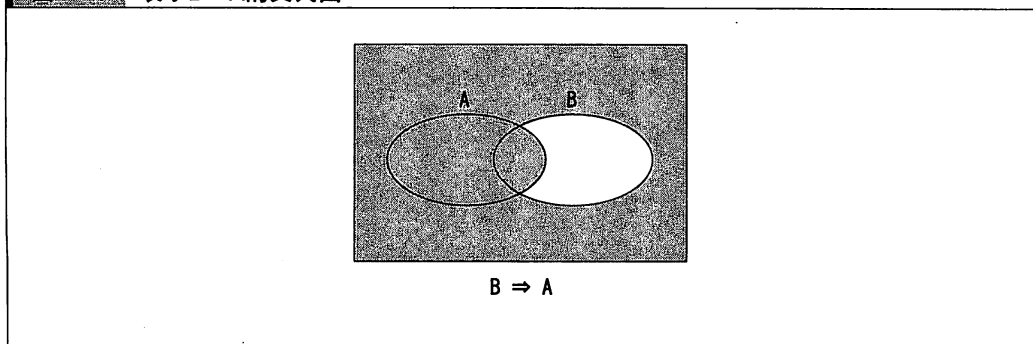
图2-23 表示 B \Rightarrow A 的文氏图
