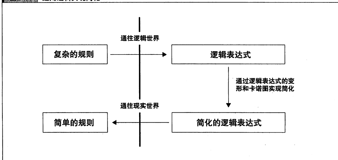
图2-39 运用逻辑实现简化
