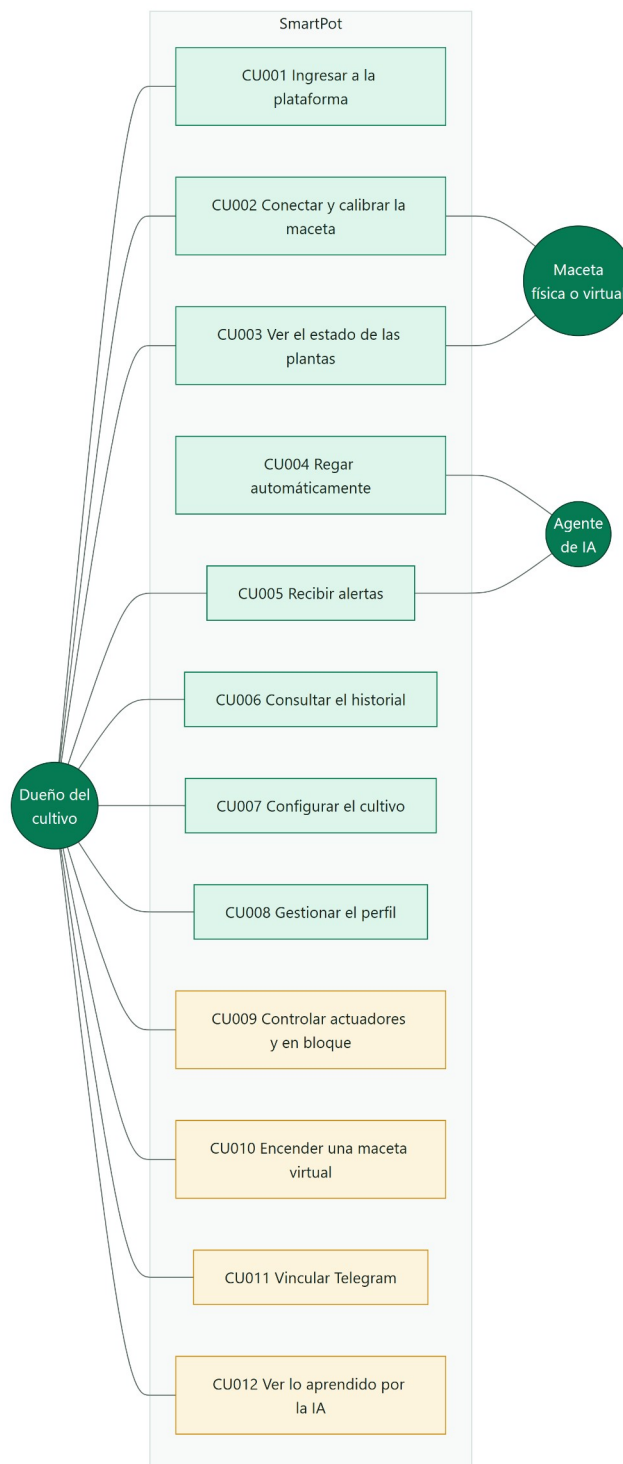
Figura 3 · Casos de uso de SmartPot
