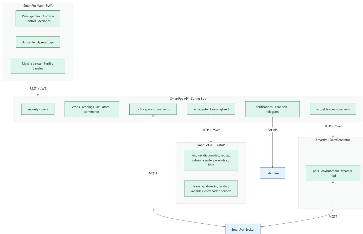
Figura 5 · Componentes y paquetes
