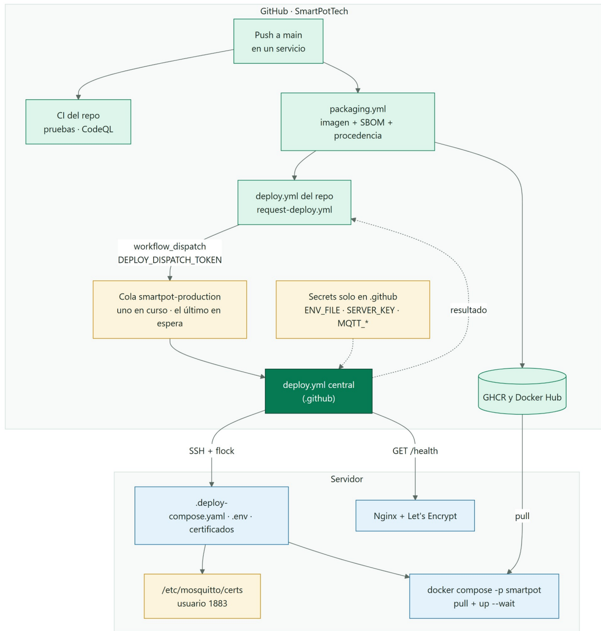
Figura 6 · Despliegue continuo
