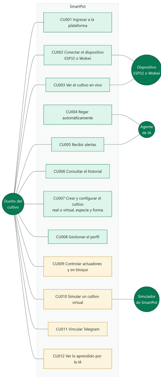
Figura 3 · Casos de uso de SmartPot
