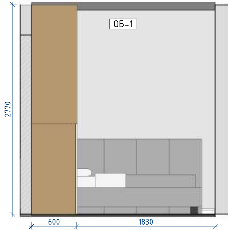
Детская 10-4 1: 30
