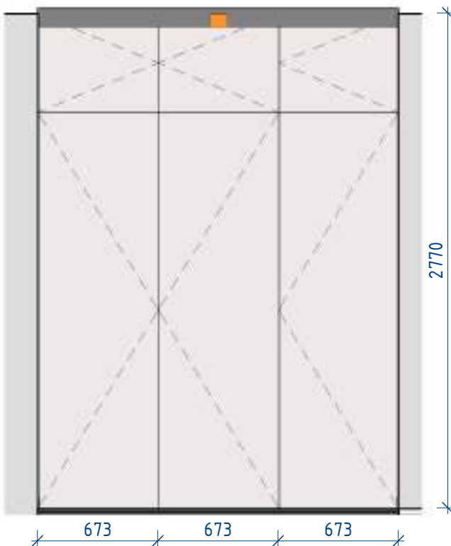
Балкон 7-2 1: 30
