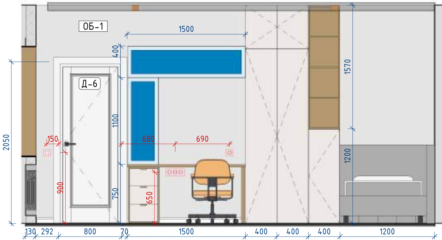
Детская 10-3 1: 30
