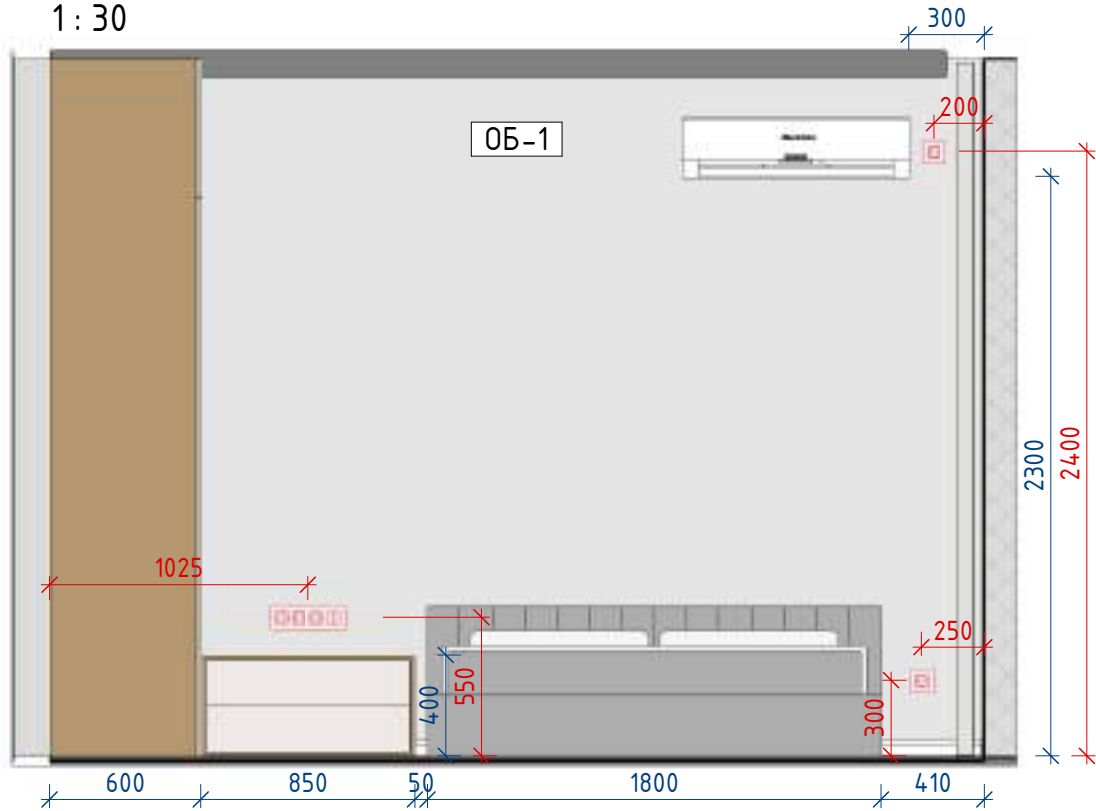
Мастер Спальня 3-3 1 : 30
