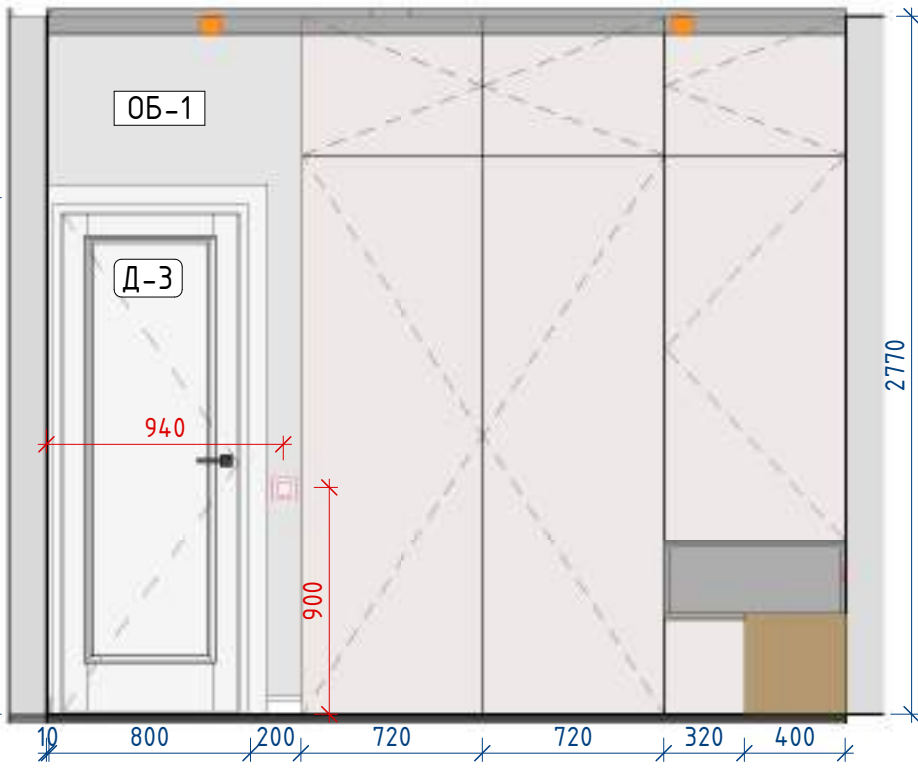
Мастер Спальня 3-4 1 : 30
