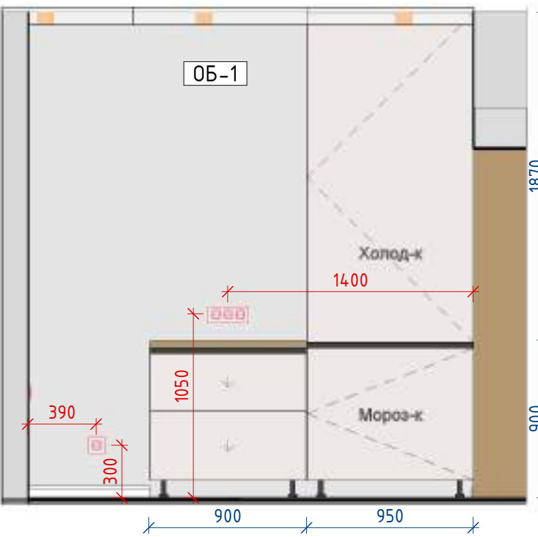
Кухня 6-4 1: 30
