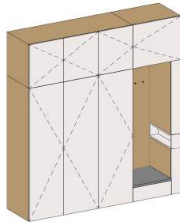
3D Шкаф коридор
