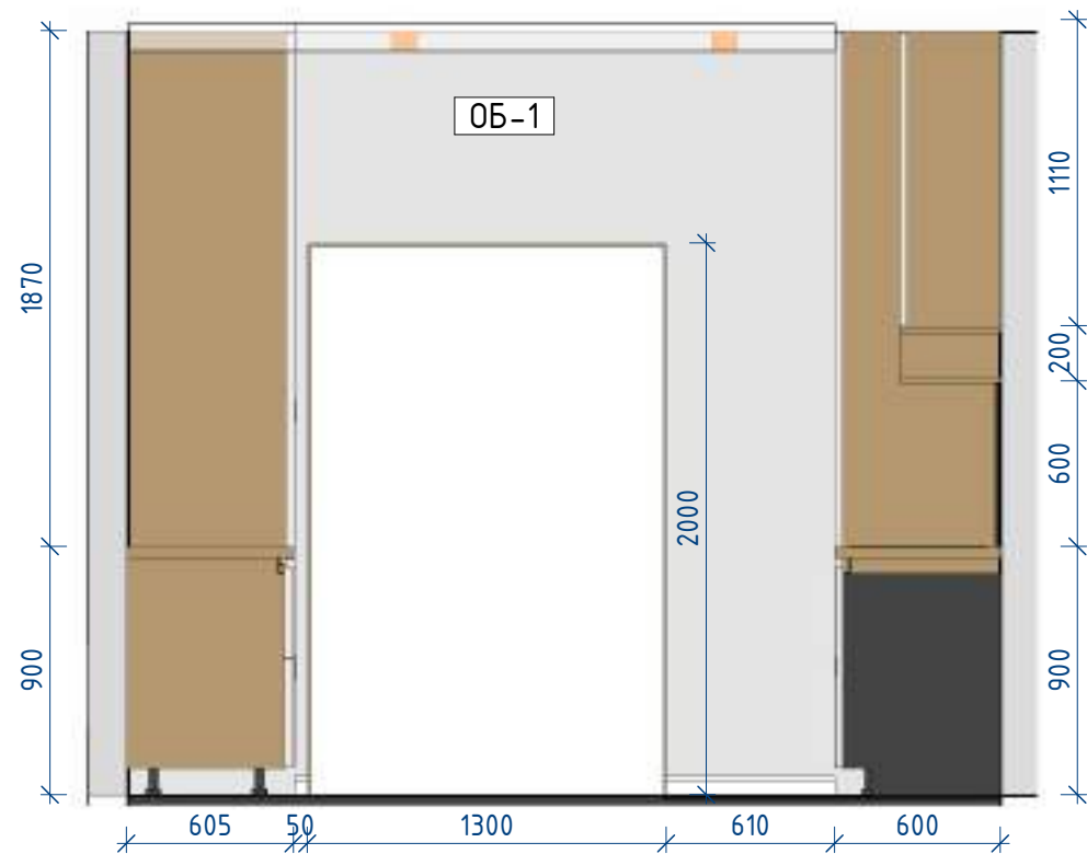
Кухня 6-1 1: 30
