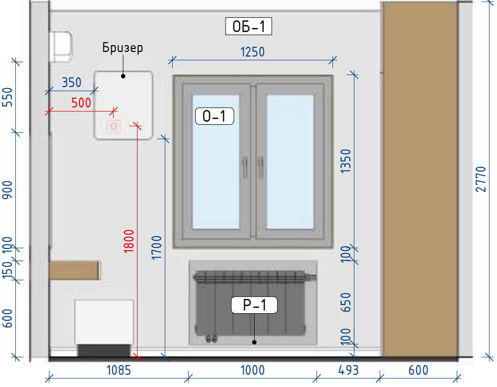
Спальня Гостевая 2-4
