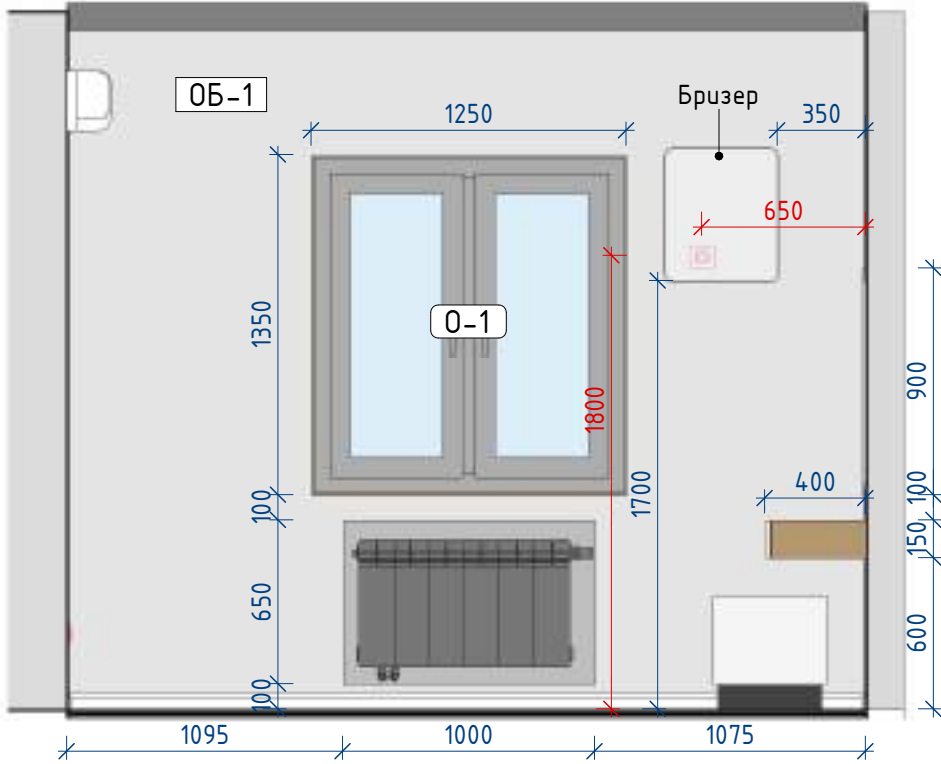
Мастер Спальня 3-2 1 : 30
