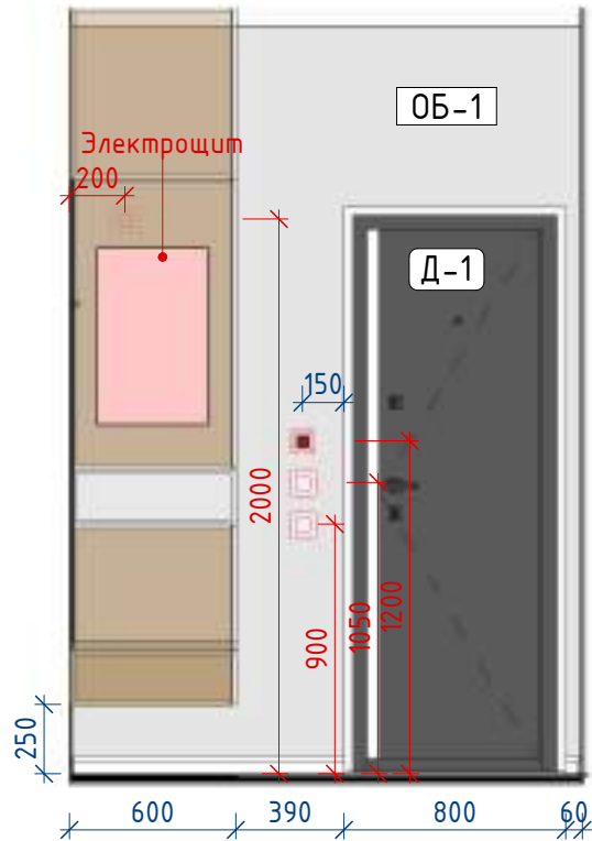
Коридор 1-1 1: 30
