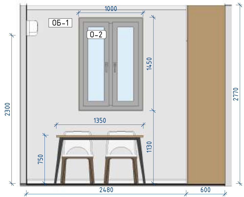
Балкон 7-1 1: 30
