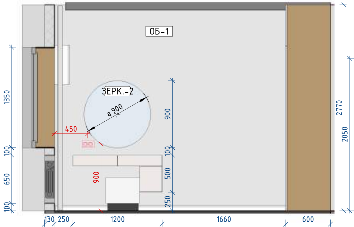
Мастер Спальня 3-3 1 : 30
