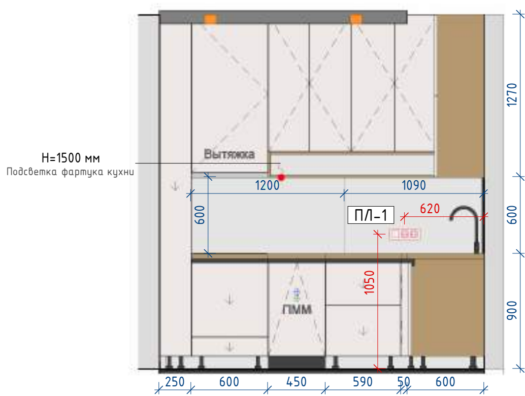
Кухня 6-2 1: 30
