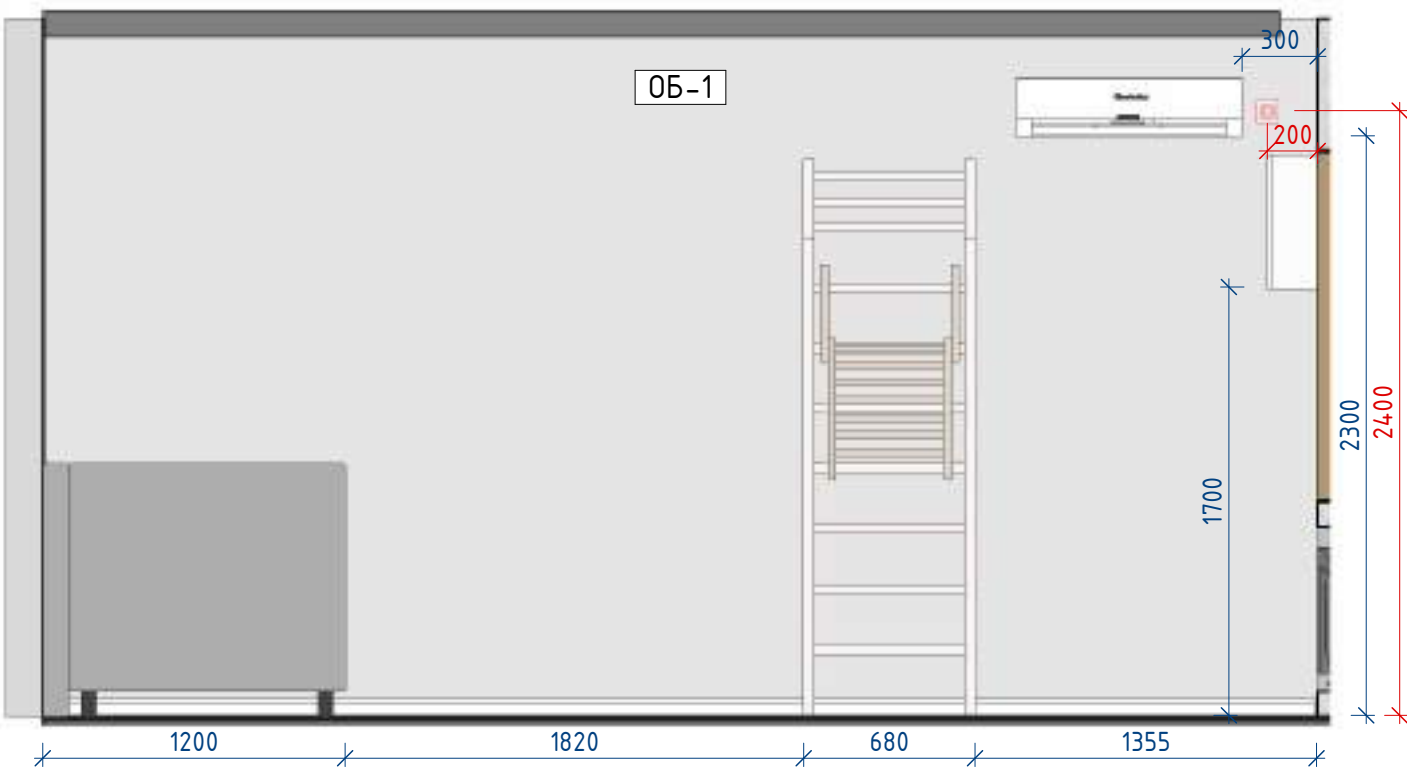
Детская 10-1 1: 30
