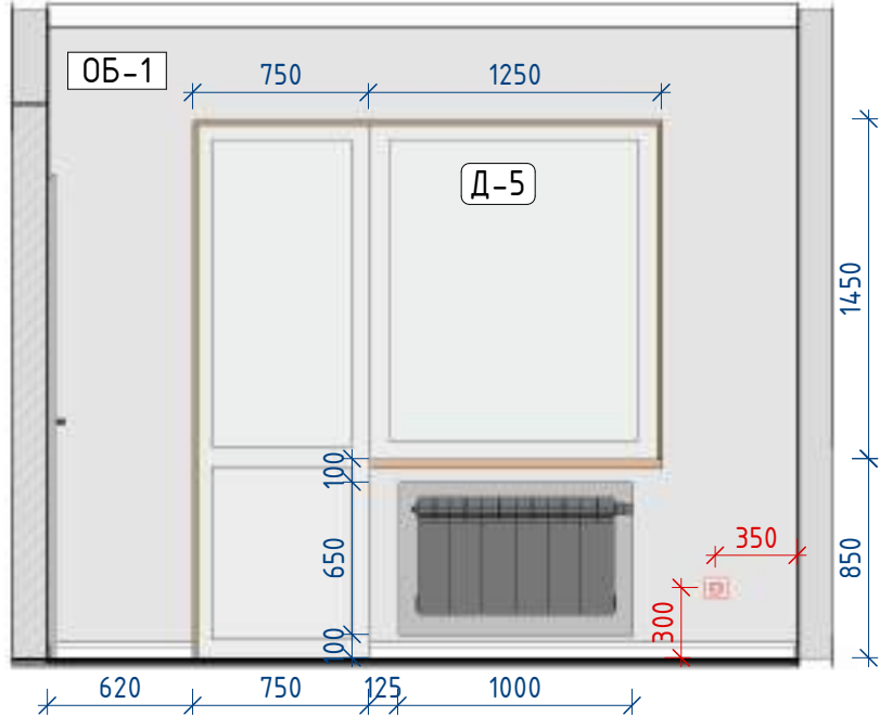
Гостиная 9-2 1: 35
