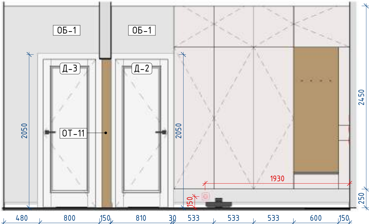
Коридор 1-4 1: 30
