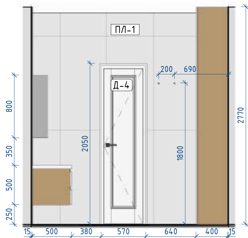
СЧ 5-1 1:30
