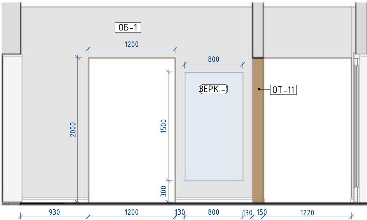
Коридор 1-2 1: 30
