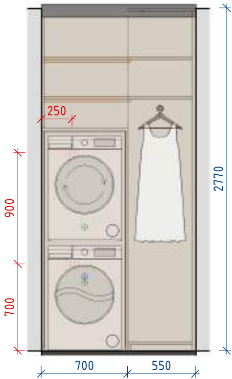
Гардероб 4-2 1:30
