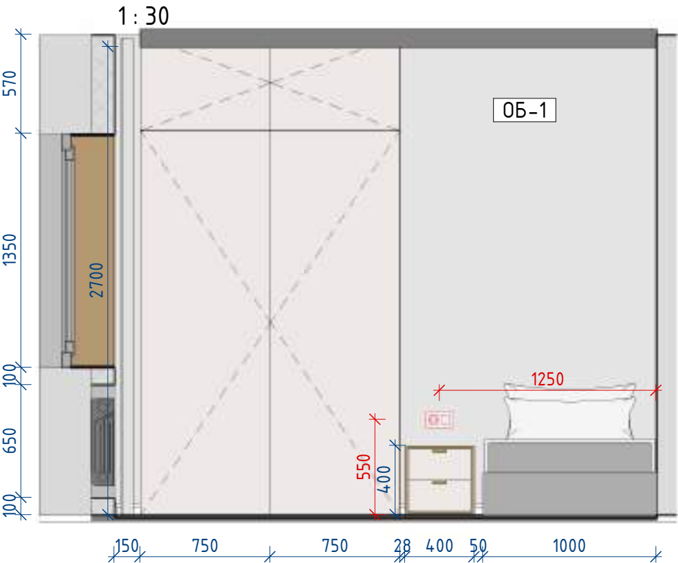
Спальня Гостевая 2-3
