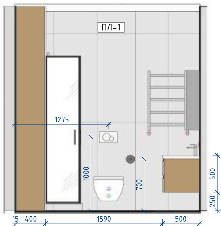
СЧ 5-3 1:30
