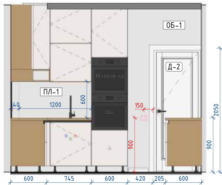
Кухня 6-3 1: 30
