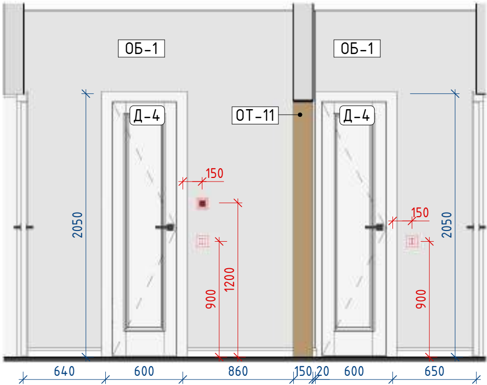
Коридор 1-3 1: 30
