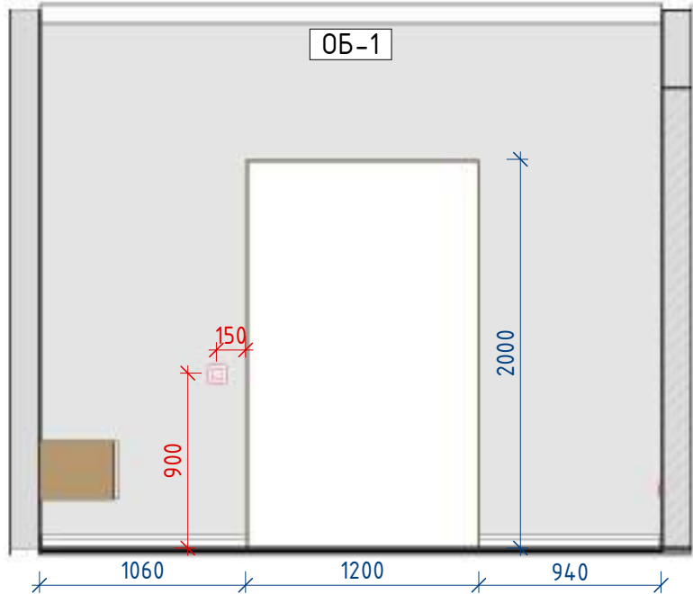
Гостиная 9-4 1: 35
