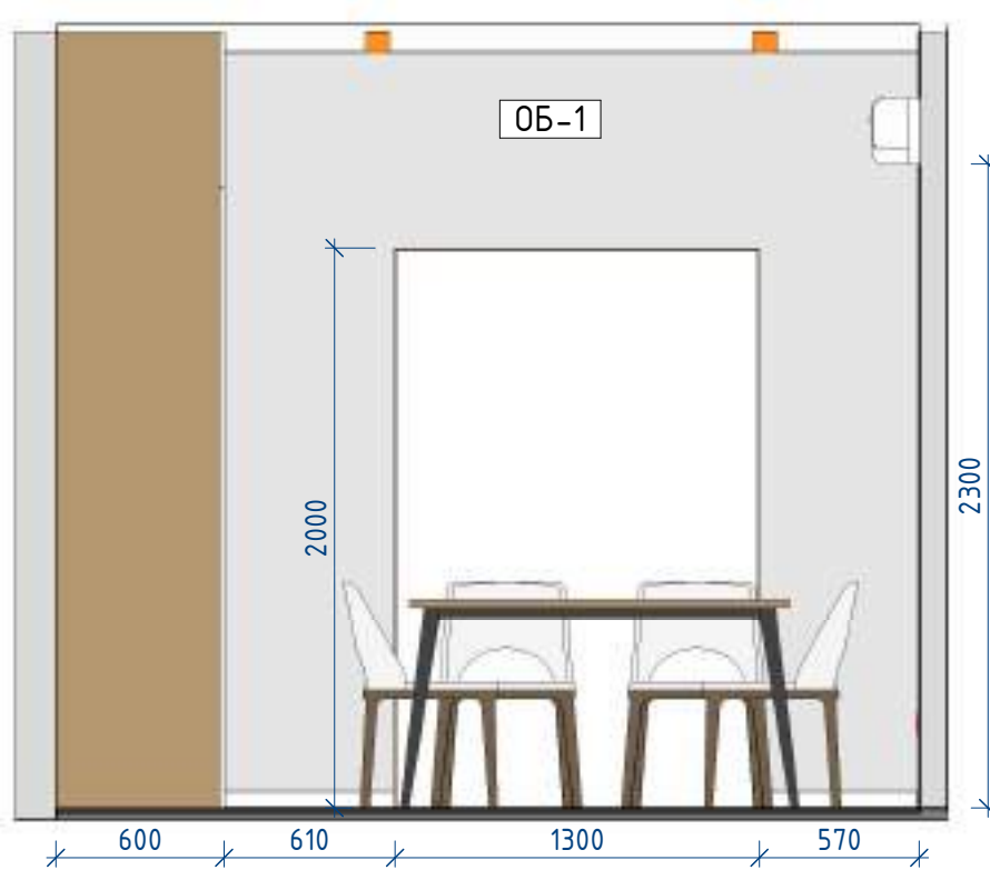
Балкон 7-3 1: 30
