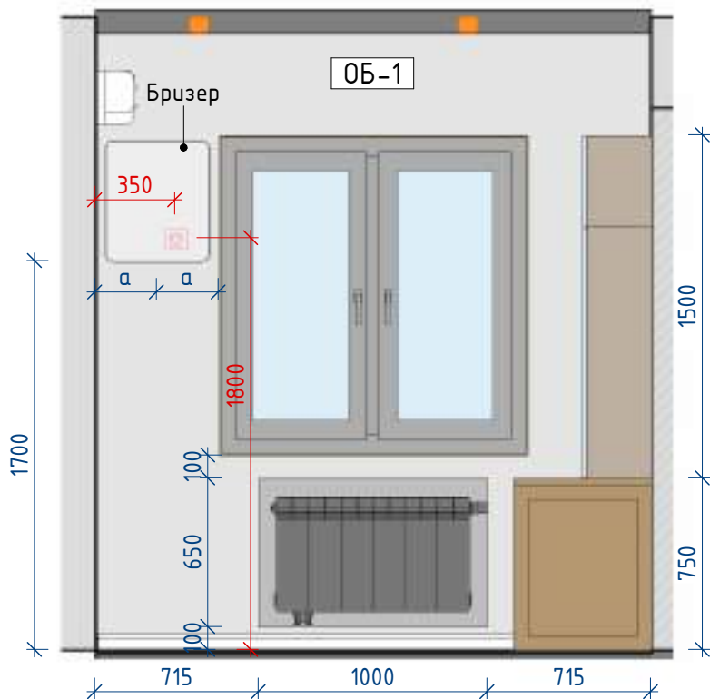
Детская 10-2 1: 30
