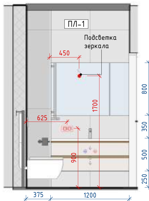
СЧ 5-4 1:30
