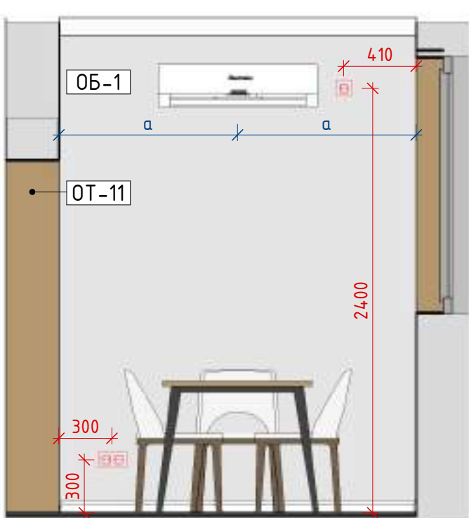
Балкон 7-4 1: 30
