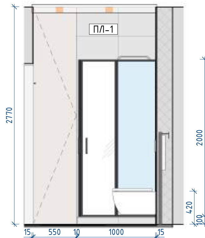
СЧ 5-2 1:30
