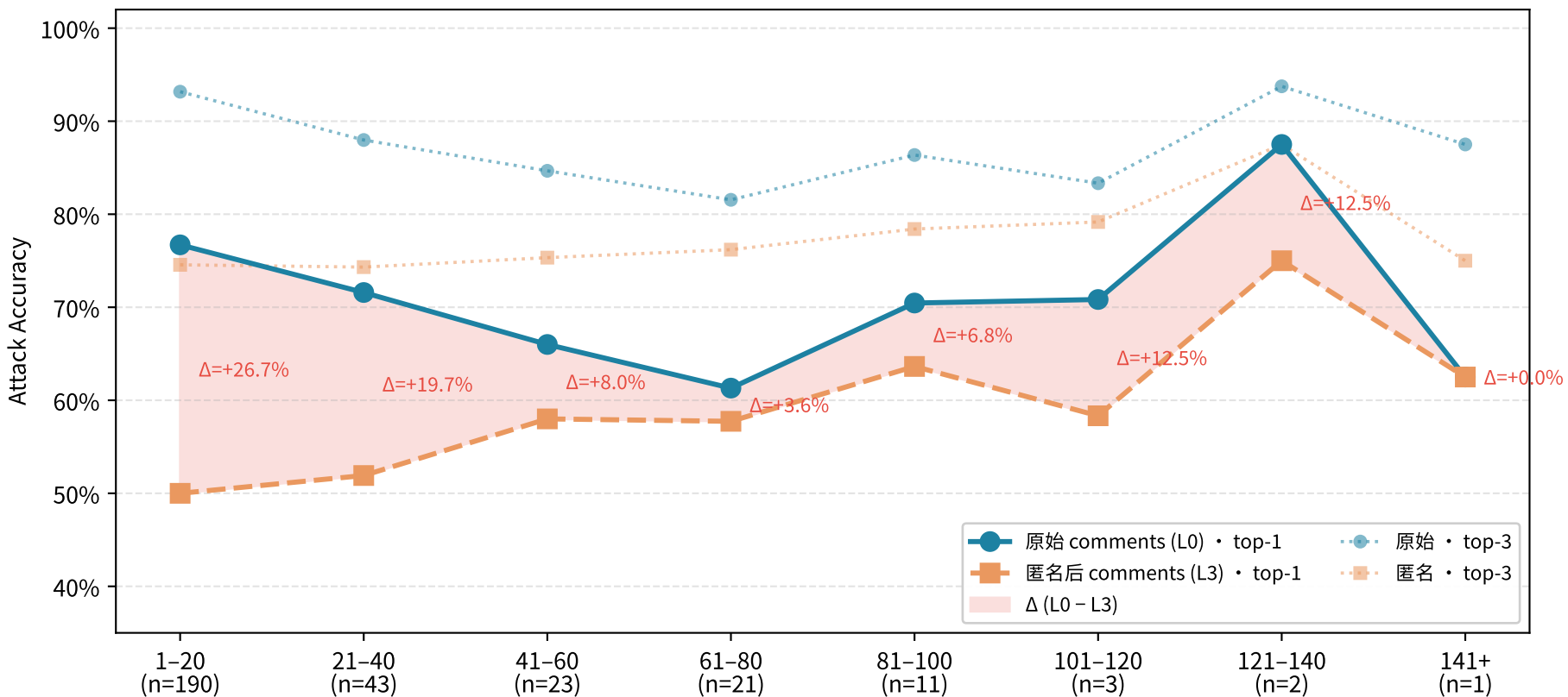
Attack Acc vs. Comment 数量 (原始 L0 vs 最后一轮匿名 L3) 合并 synthpai 250pers + remaining 50pers • deepseek-chat-full-comments • micro-avg
