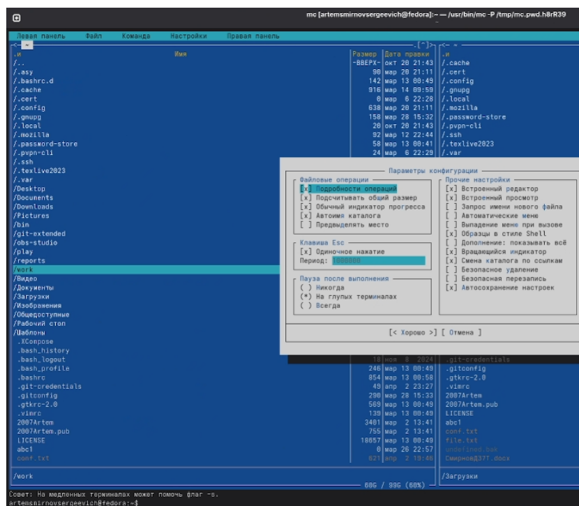
Рис. 4.17: Диалог «Конфигурация»
