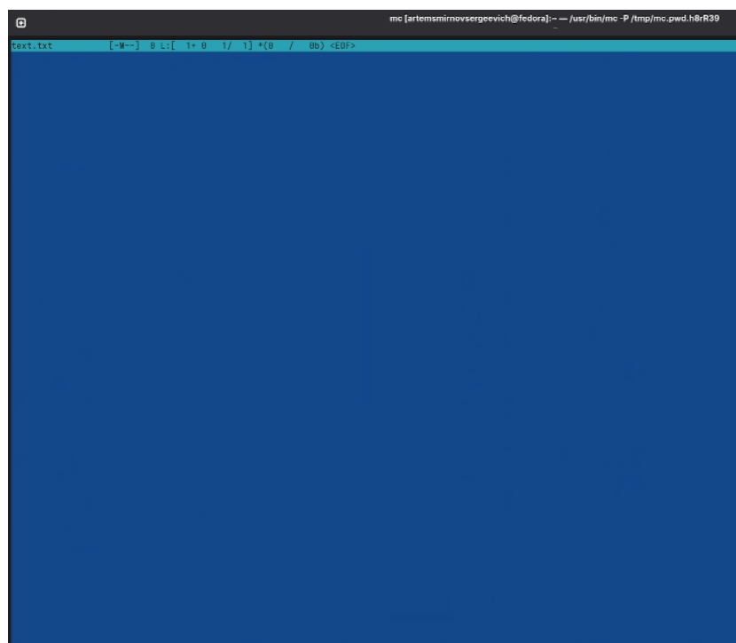
Рис. 4.20: Редактирование текста
