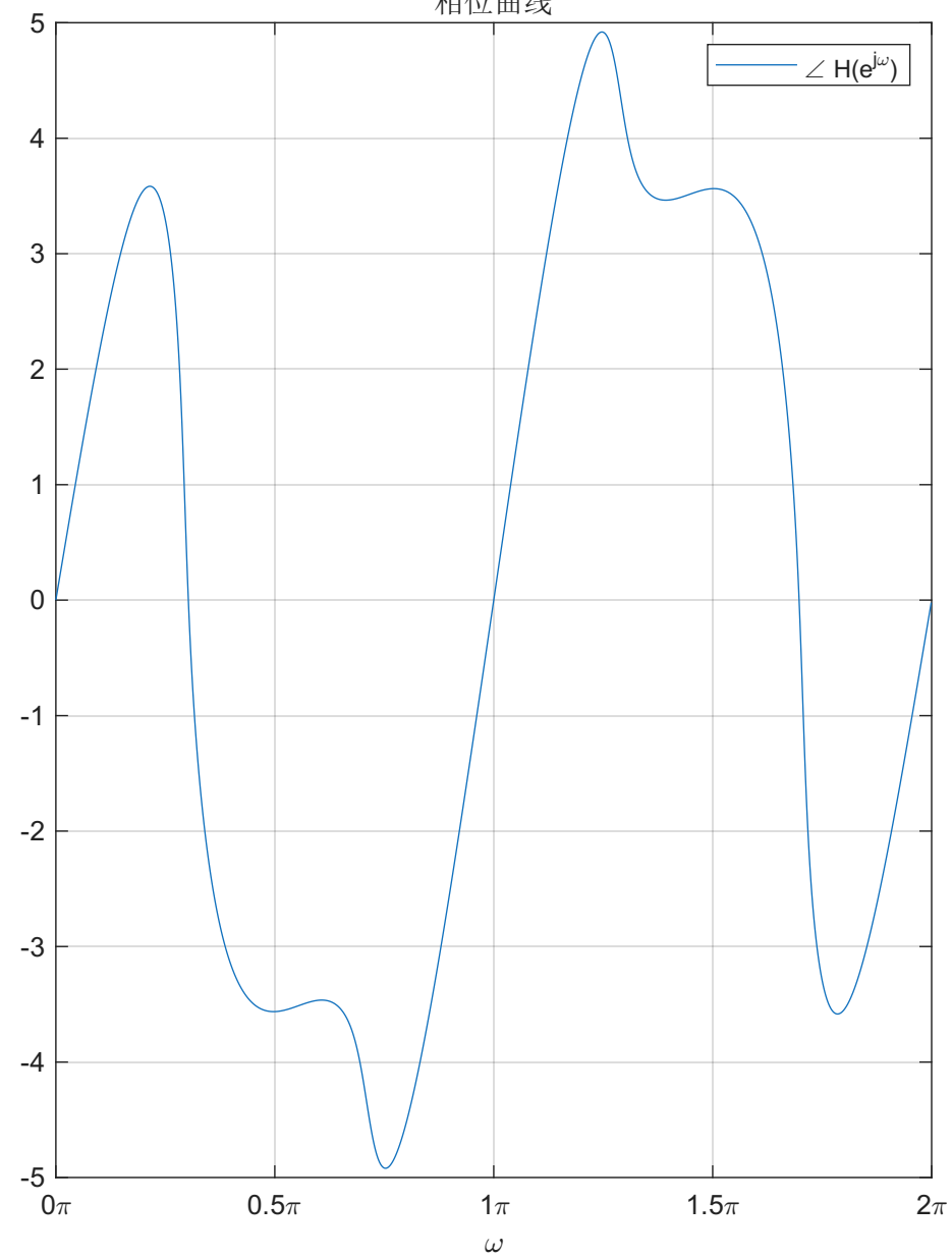
相位曲线
