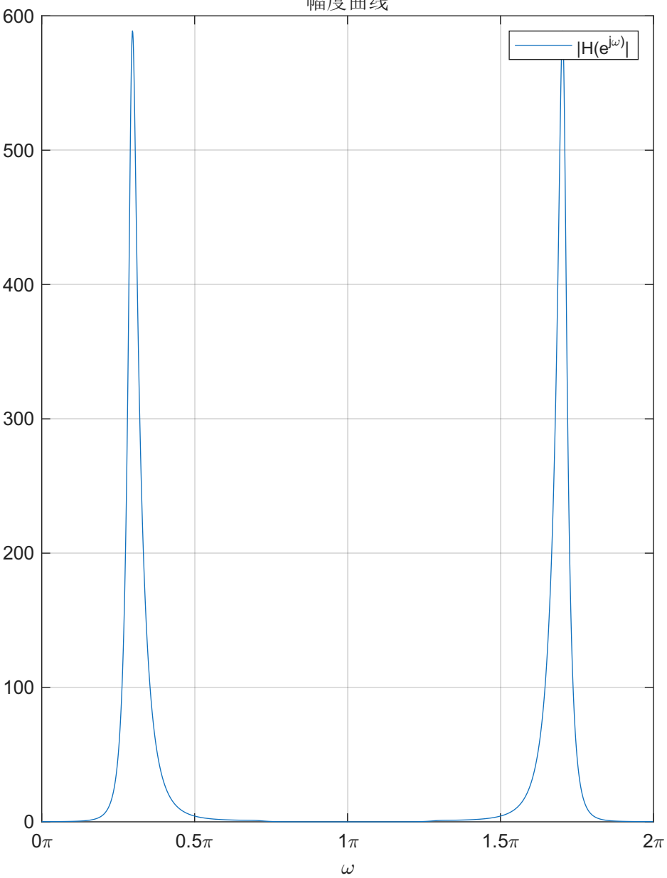
幅度曲线
