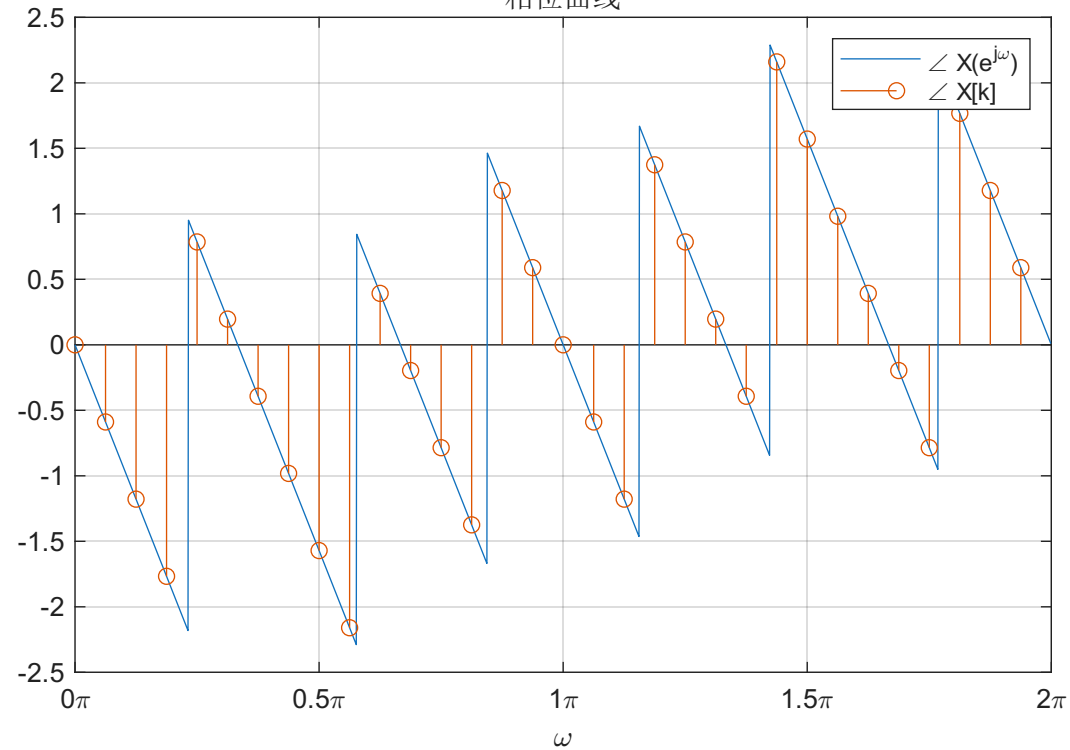
相位曲线
