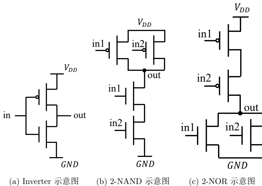
图 1: Inverter, 2-NAND, 2-NOR 示意图
