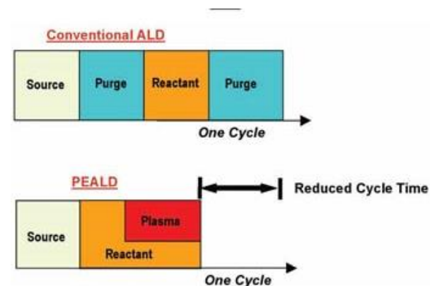
热ALD与等离子体增强ALD的比较
