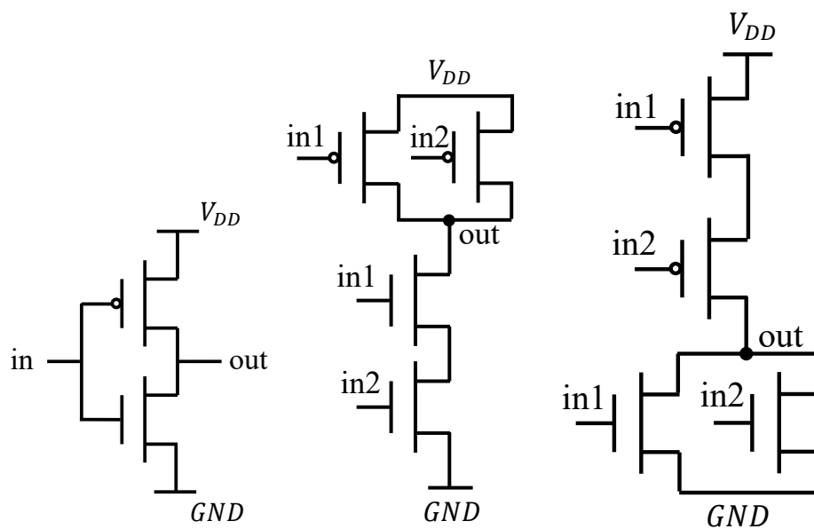
(a) Inverter 示意图 (b) 2-NAND 示意图 (c) 2-NOR 示意图
