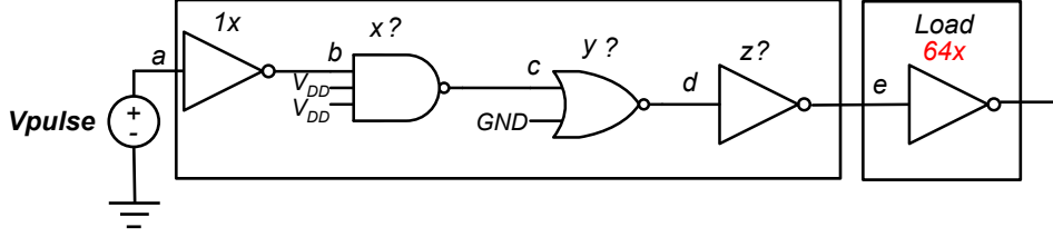
图 3: Task1 电路
