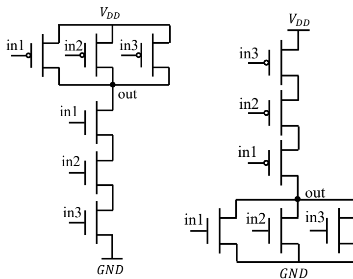
(a) 3-NAND 示意图 (b) 3-NOR 示意图
