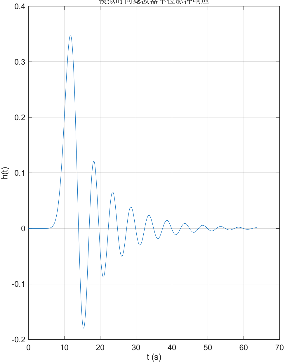
模拟时间滤波器单位脉冲响应
