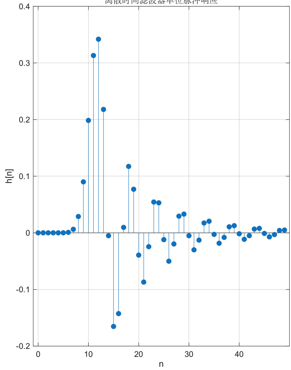
离散时间滤波器单位脉冲响应
