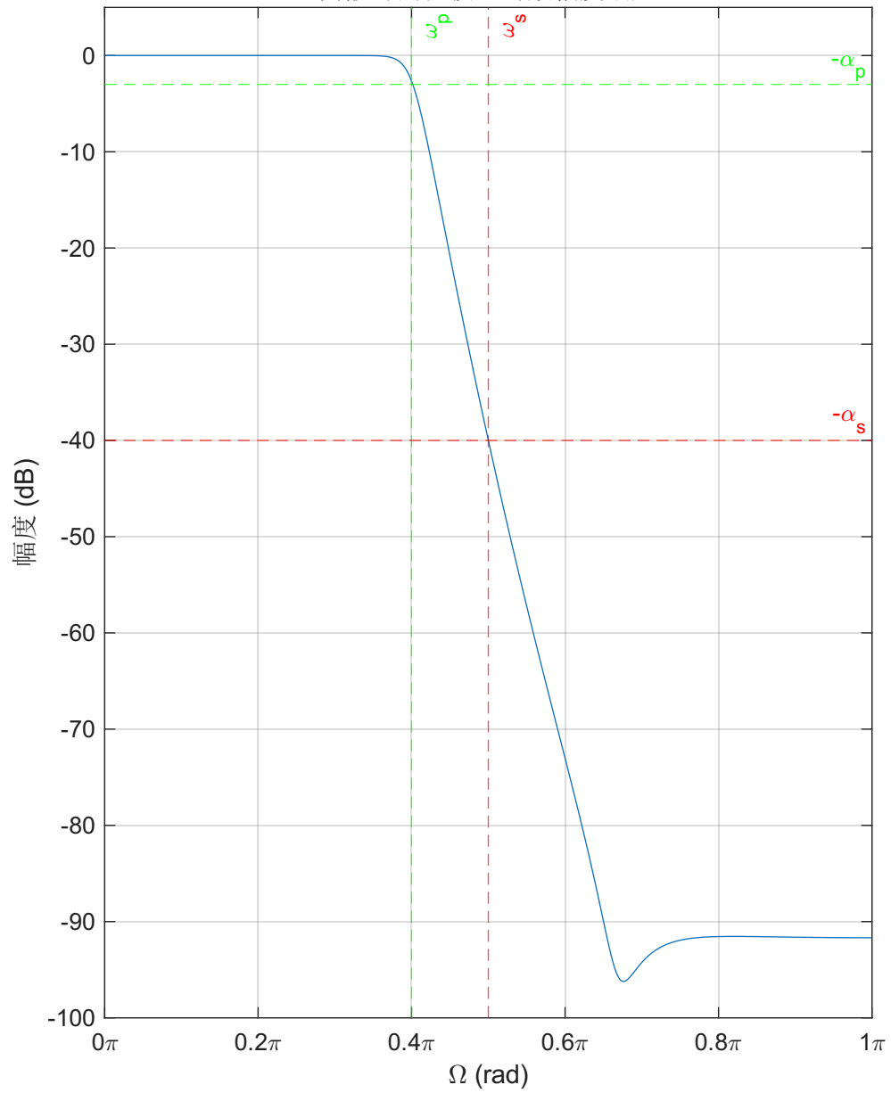
离散时间滤波器对数幅度响应
