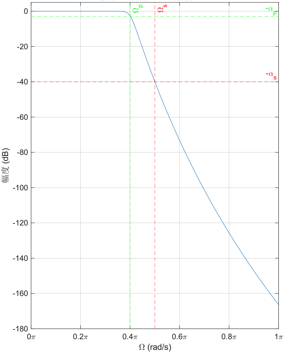
模拟时间滤波器对数幅度响应
