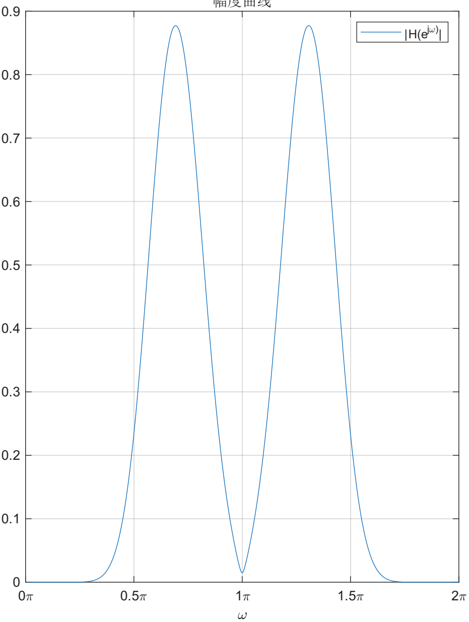
幅度曲线
