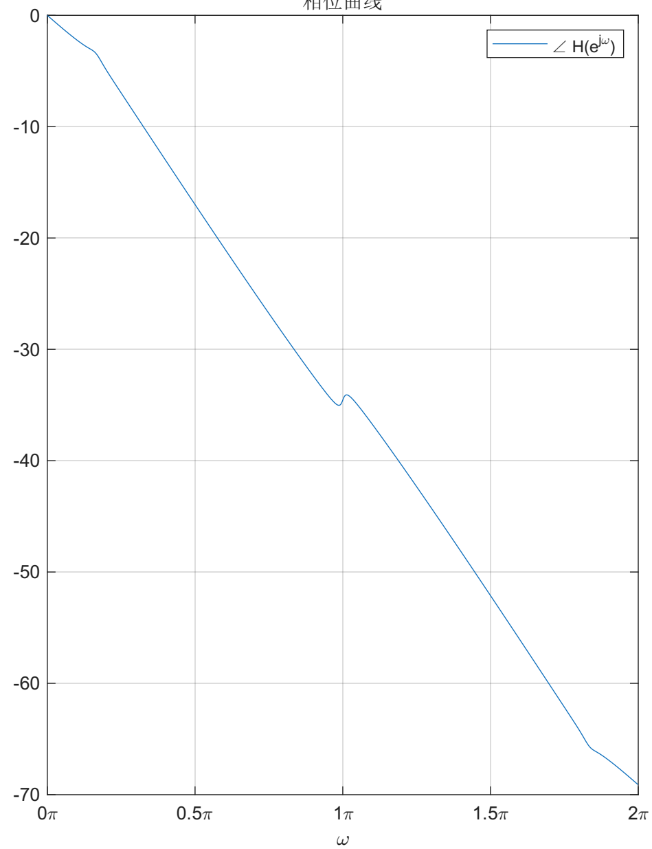
相位曲线
