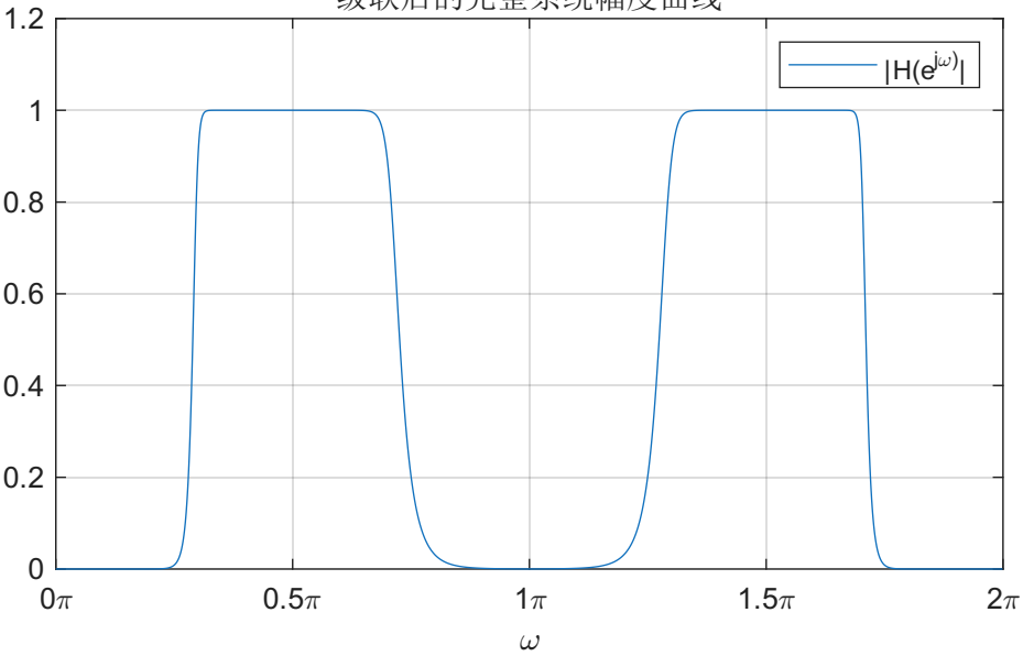
级联后的完整系统幅度曲线
