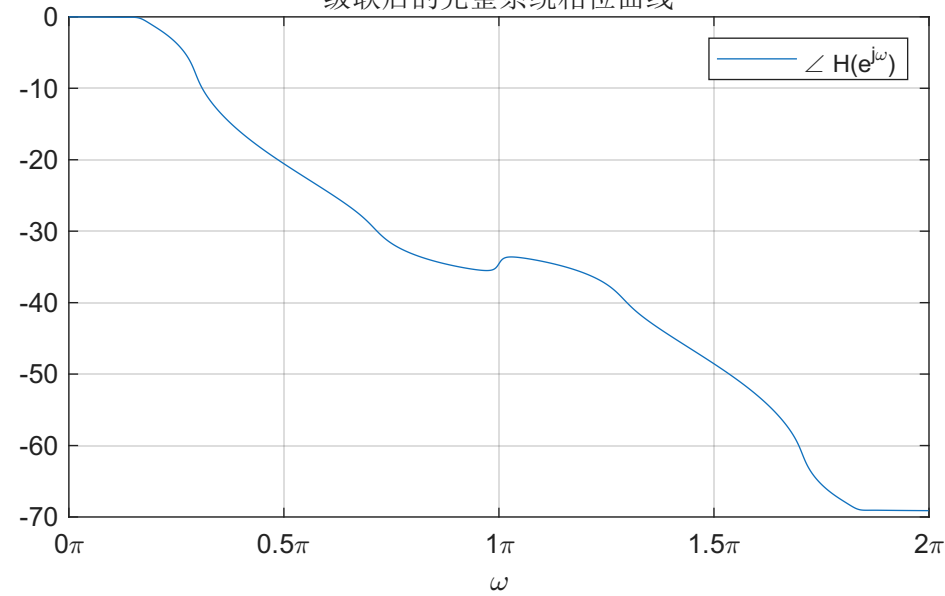
级联后的完整系统相位曲线
