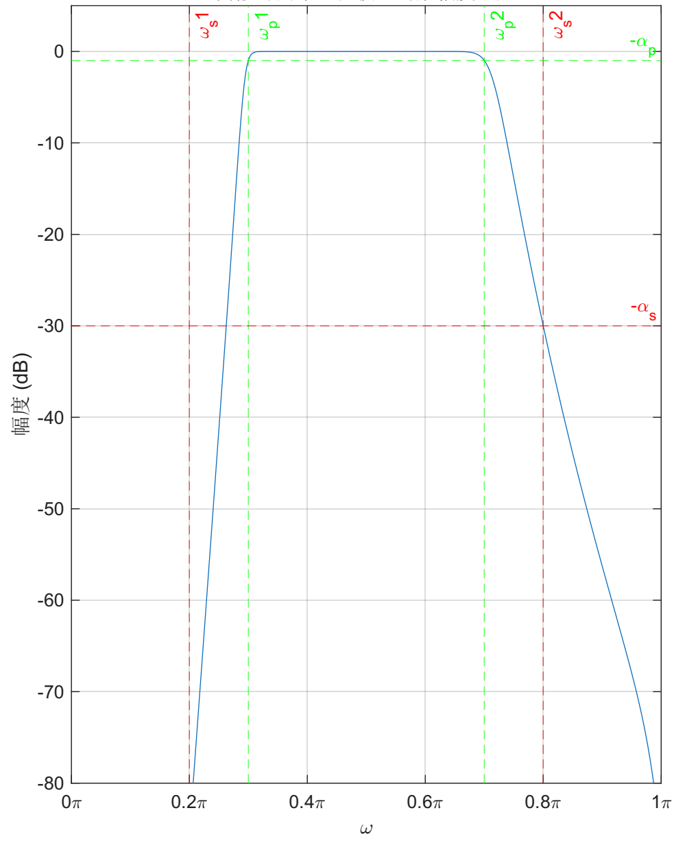
离散时间带通滤波器对数幅度响应
