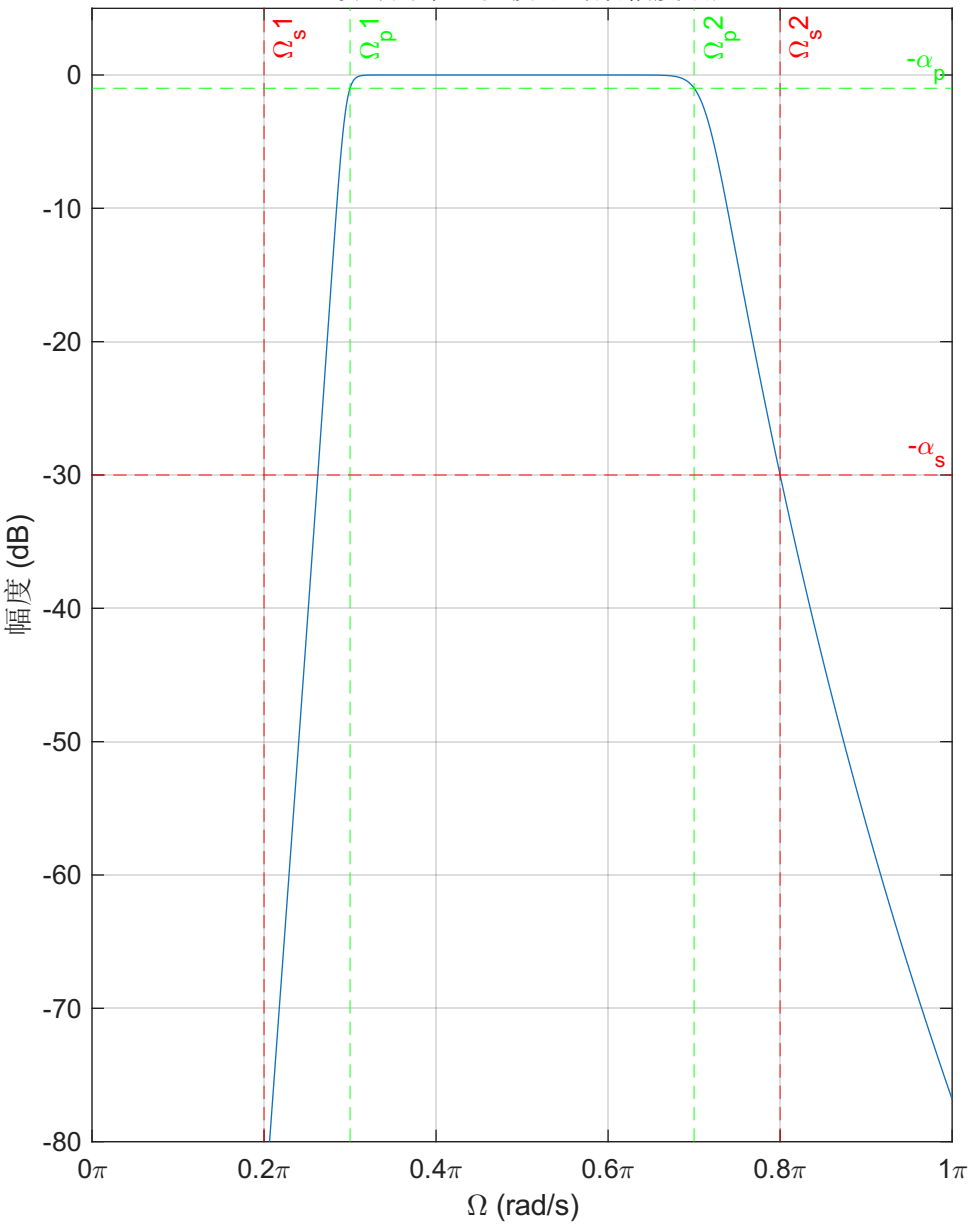
连续时间带通滤波器对数幅度响应
