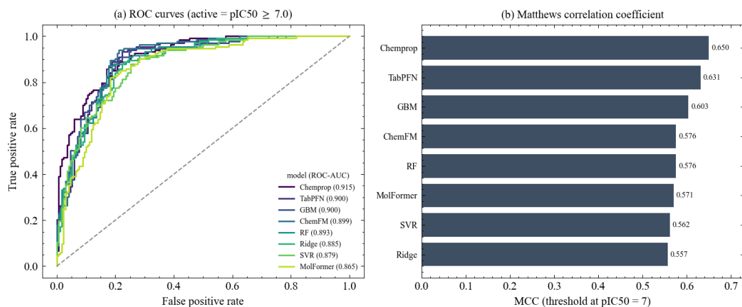
图 18 分类视角：(a) 8 个模型的 ROC 曲线（active = pIC 50 ≥ 7.0）；(b) MCC：Chemprop 最高，回归最优的 TabPFN 在分类轴略逊
