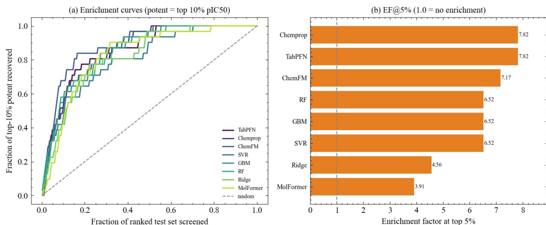
图 19 早期富集（高活性 = 最高 10%，pIC 50 ≥ 8.04）：(a) 富集曲线；(b) EF@5%：各模型在排序表头富集约 4–7 倍于随机
