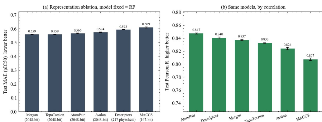
图 15 表征消融（模型固定为随机森林）：(a) 测试 MAE；(b) 测试 Pearson R：Morgan / Atom Pair / Topological Torsion 同属第一梯队，MACCS 最弱
