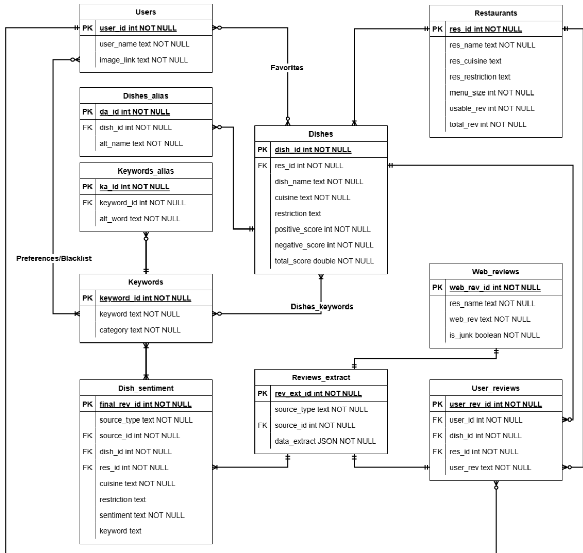
Figure 3.9: ER Diagram
