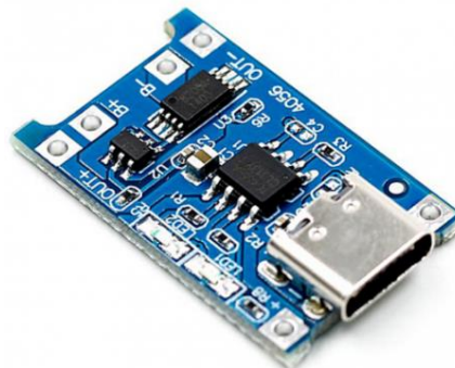
Fig 3.2 TP4056 Li-ion
