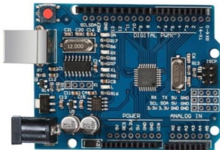
Fig 3.1 Arduino Uno R3
