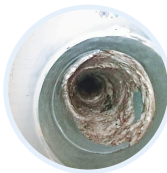
Vue caméra dans une canalisation
